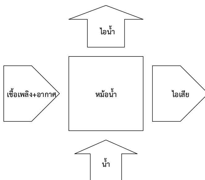
รูปที่ 4.9 แผนผังการประเมินประสิทธิภาพหม้อน้ำด้วยวิธีทางตรง
