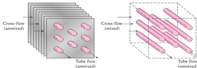
รูปที่ 7.9 หลักการแลกเปลี่ยนความร้อนของเครื่องแลกเปลี่ยนความร้อนแบบของไหลมีทิศทางตั้งฉากกัน
