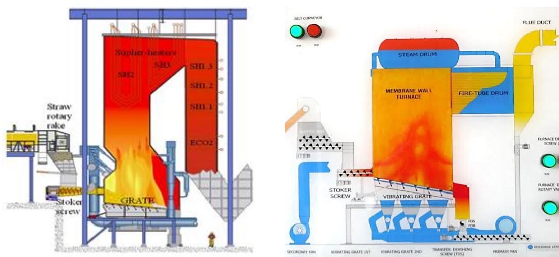
รูปที่ 3.11 ตะกรับเตาสั่นสะเทือน (Vibrating grate)
