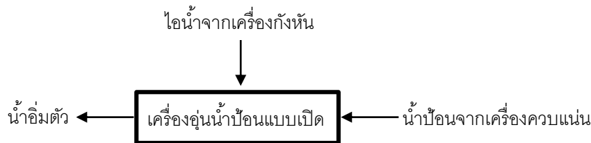
รูปที่ 2.4 เครื่องอุ่นน้ำป้อนแบบเปิด
