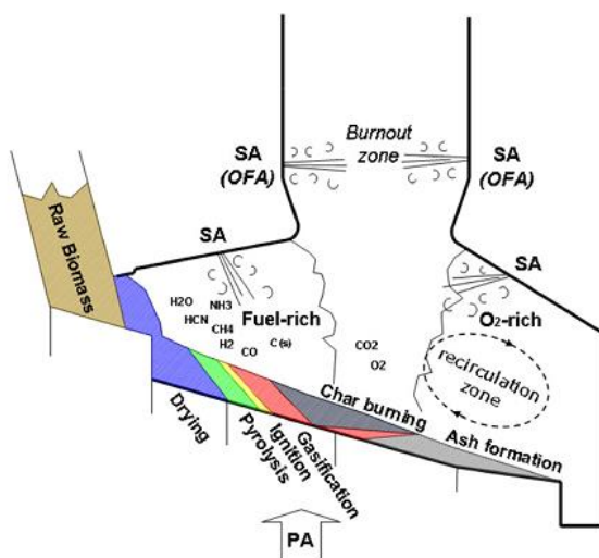
รูปที่ 3.8 ตะกรับไฟเอียงอยู่กับที่ (Stationary sloping grate)
