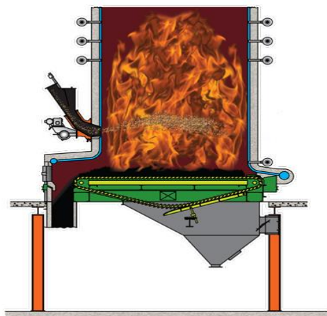
รูปที่ 3.9 ตะกรับเตาเคลื่อนที่ (Travelling grate)
