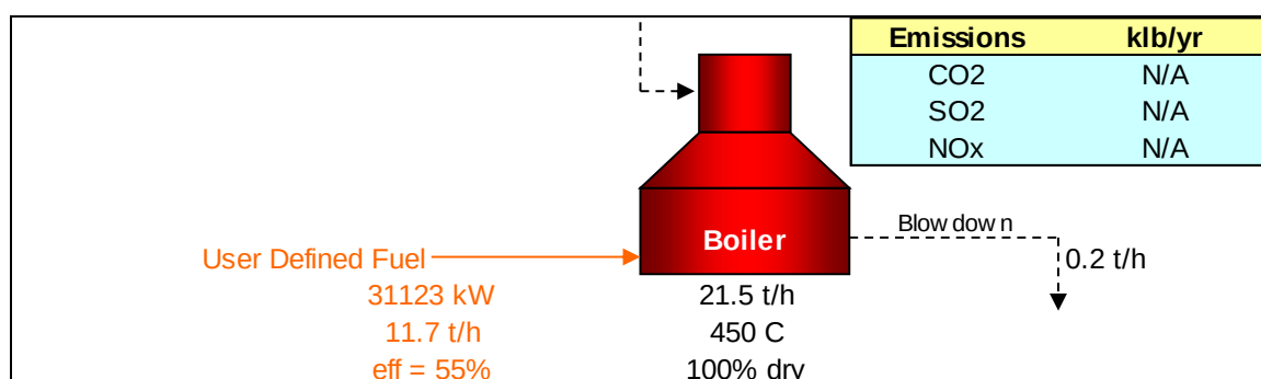
รูปที่ 9.39 แบบจำลองจากการลดการสูญเสียเนื่องจากการรั่วไหลของอากาศที่เข้าสู่ระบบก๊าซไอเสียของหม้อน้ำด้วยโปรแกรม SSAT
