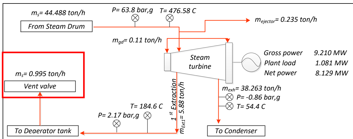
รูปที่ 9.40 ไดอะแกรมการใช้ไอน้ำ ณ วันที่เข้าตรวจวัดกังหันไอน้ำ (ก่อนปรับปรุง)
