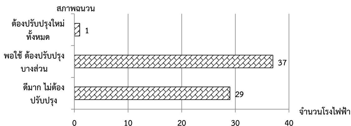
รูปที่ 1.16 สภาพฉนวนในระบบท่อส่งจ่ายไอน้ำของโรงไฟฟ้าชีวมวลขนาดเล็กมาก (ข้อมูลจากแบบสอบถาม 70 โรงไฟฟ้า)
