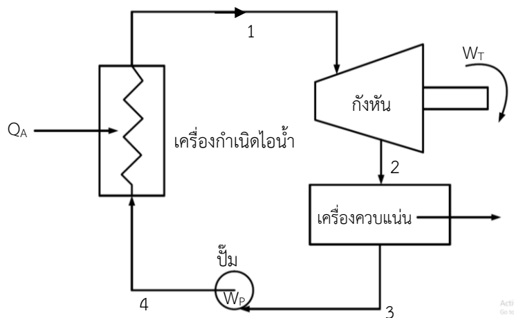
รูปที่ 2.2 แผนภาพการทำงานอย่างง่ายของวัฏจักรแรงคิน
