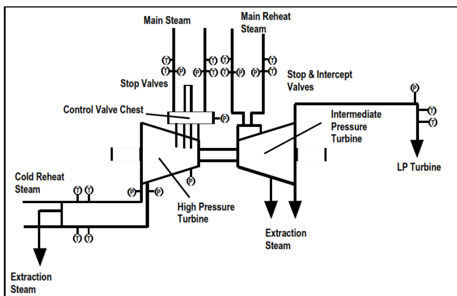
รูปที่ 6.12 ตำแหน่งการวัดทั้งหมด
