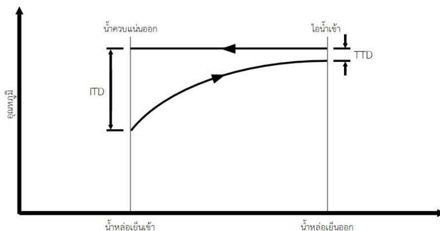
รูปที่ 7.7 โพรไฟล์อุณหภูมิในเครื่องควบแน่นผิวสัมผัส
