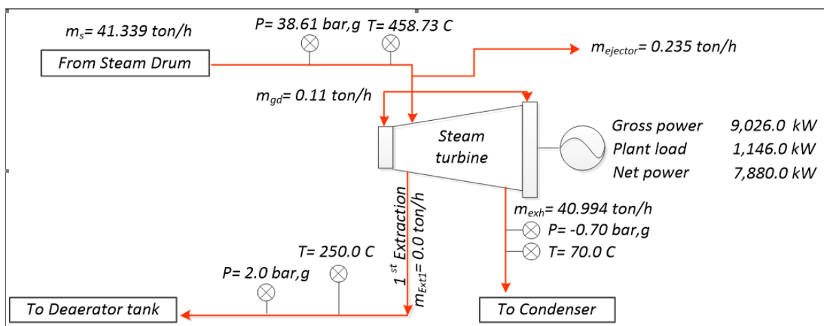
รูปที่ 6.24 ไดอะแกรมการใช้ไอน้ำของกังหันไอน้ำ (Steam turbine)
