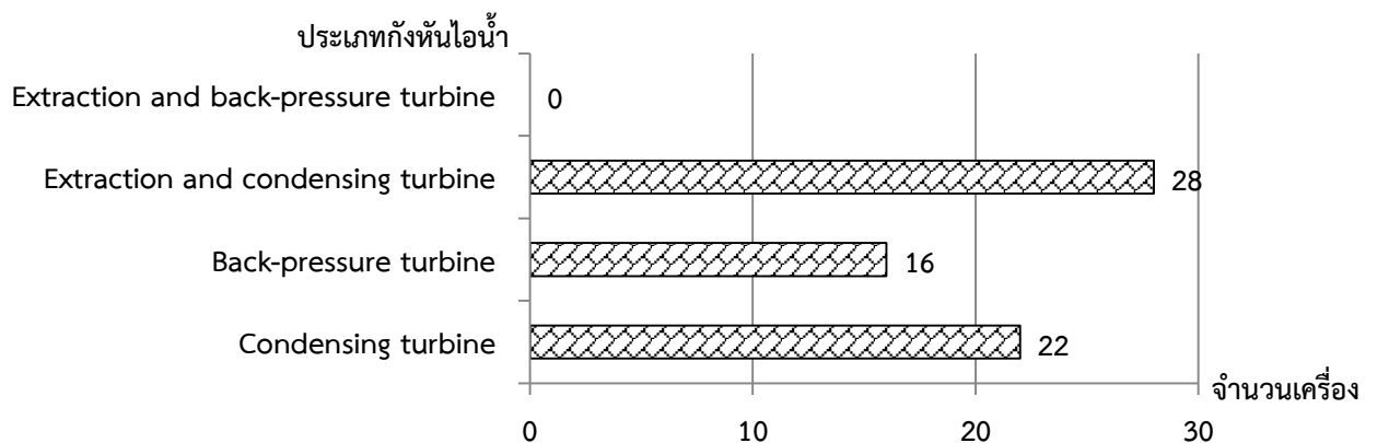
รูปที่ 1.19 ประเภทของกังหันไอน้ำที่ใช้ในโรงไฟฟ้าชีวมวลขนาดเล็กมาก (ข้อมูลจากแบบสอบถาม 70 โรงไฟฟ้า)
