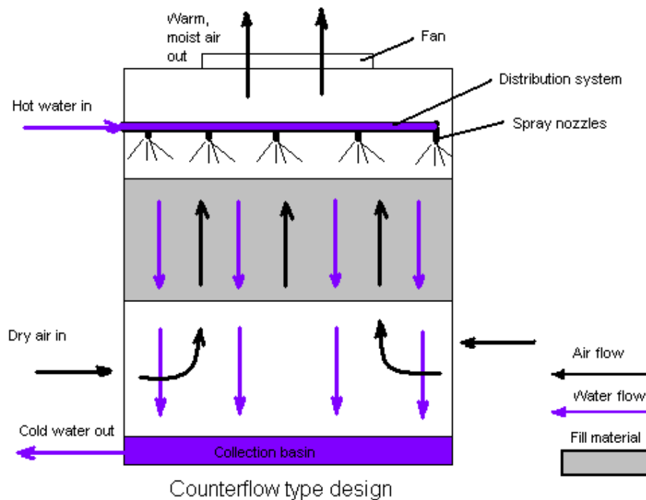
(ข) แผนภาพหอผึ่งเย็นแบบไหลสวนทาง
