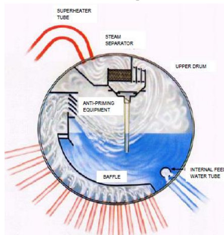
รูปที่ 4.5 (ข) การแยกไอน้ำโดยวิธีต่างๆ ในถังพักไอน้ำ แบบเชิงกล (Mechanic)
