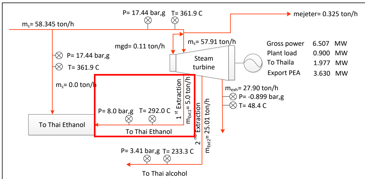
รูปที่ 9.72 ไดอะแกรมการใช้ไอน้ำหลังปรับปรุงมาตรการนำไอน้ำส่งให้เอทานอลที่ 8 barg มาผ่านกังหันไอน้ำ
