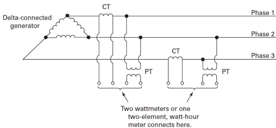
รูปที่ 6.10 การวัดกำลังไฟฟ้า แบบ Three-Wire System (Delta)
