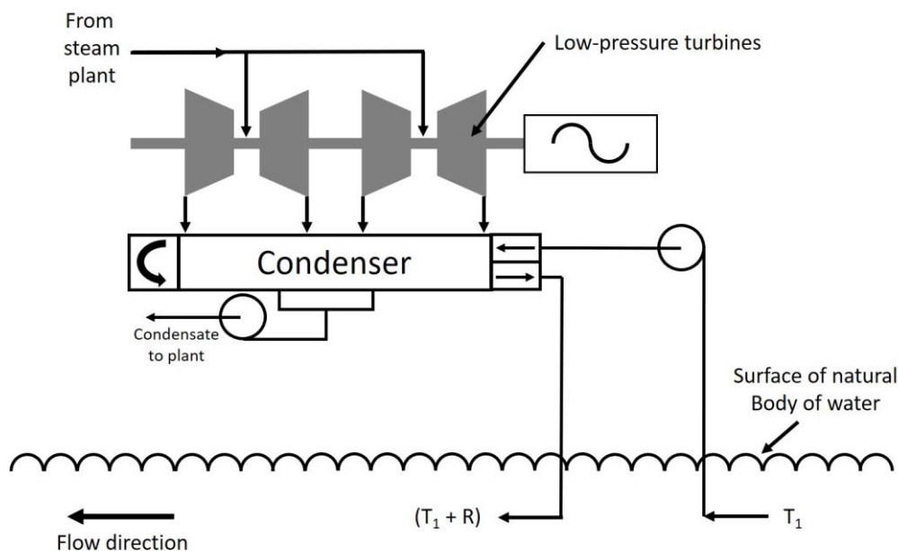
รูปที่ 8.1 ระบบน้ำหล่อเย็นแบบเปิด
