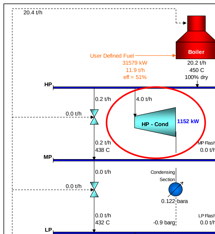
รูปที่ 9.66 แบบจำลองจากมาตรการเพิ่มกำลังการผลิตไฟฟ้า
