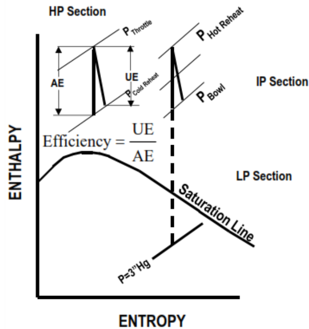
รูปที่ 6.13 การหาประสิทธิภาพของกังหันไอน้ำโดยใช้ Entropy drop test
