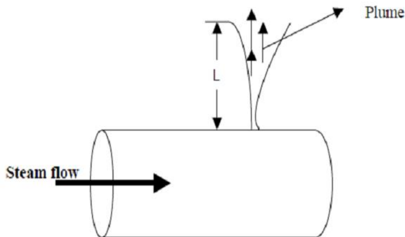
รูปที่ 5.6 การวัดความยาวการฟุ้งกระจายตัวของกลุ่มไอน้ำ (plume length)
