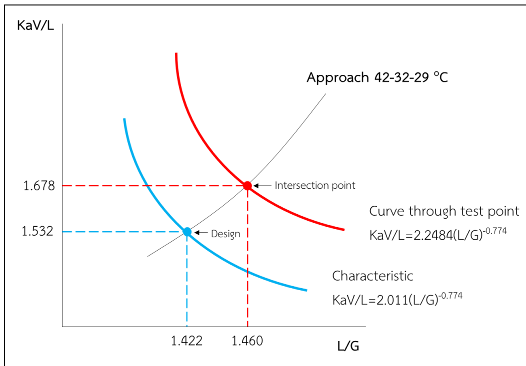
รูปที่ 8.9 กราฟ Tower Demand & Characteristic Curves
