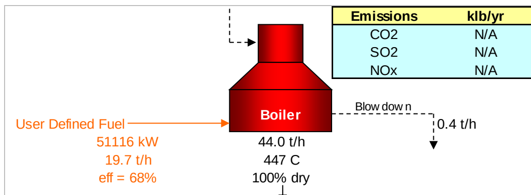
รูปที่ 9.25 แบบจำลองจากการปรับแต่งการเผาไหม้ของหม้อน้ำด้วยโปรแกรม SSAT
