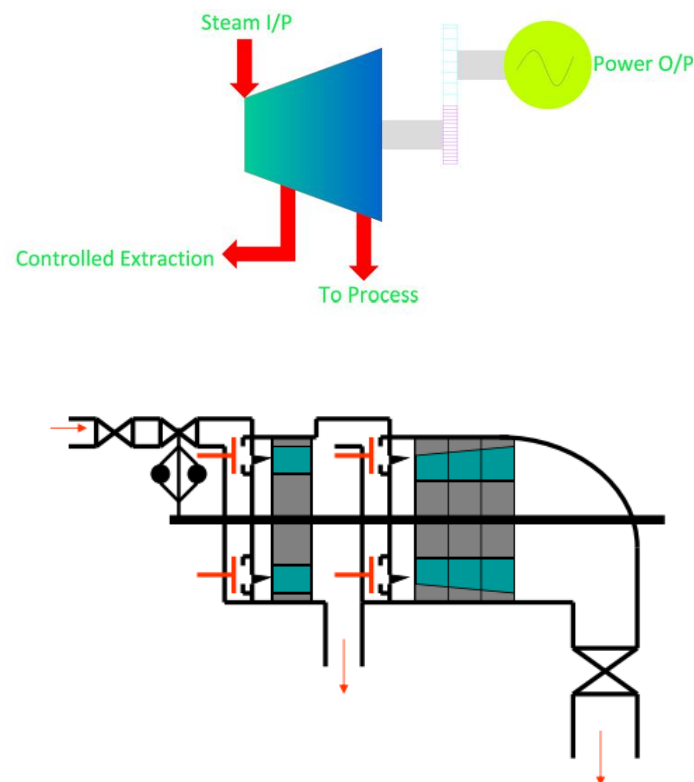
รูปที่ 6.4 แผงผังของ Back pressure extraction turbine
