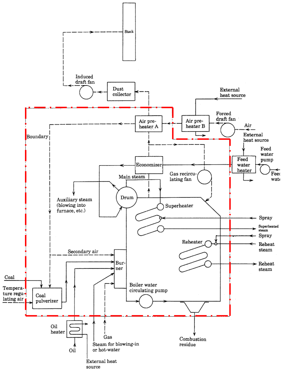
รูปที่ 4.11 ขอบเขตของการทำสมดุลพลังงานความร้อนในหม้อน้ำในกรอบสีแดง
