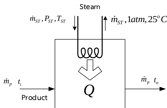
รูปที่ 7.11 แสดงหลักการคำนวณประสิทธิภาพการแลกเปลี่ยนความร้อน
