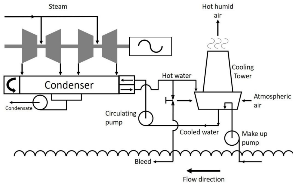
รูปที่ 8.2 ระบบน้ำหล่อเย็นแบบปิด
