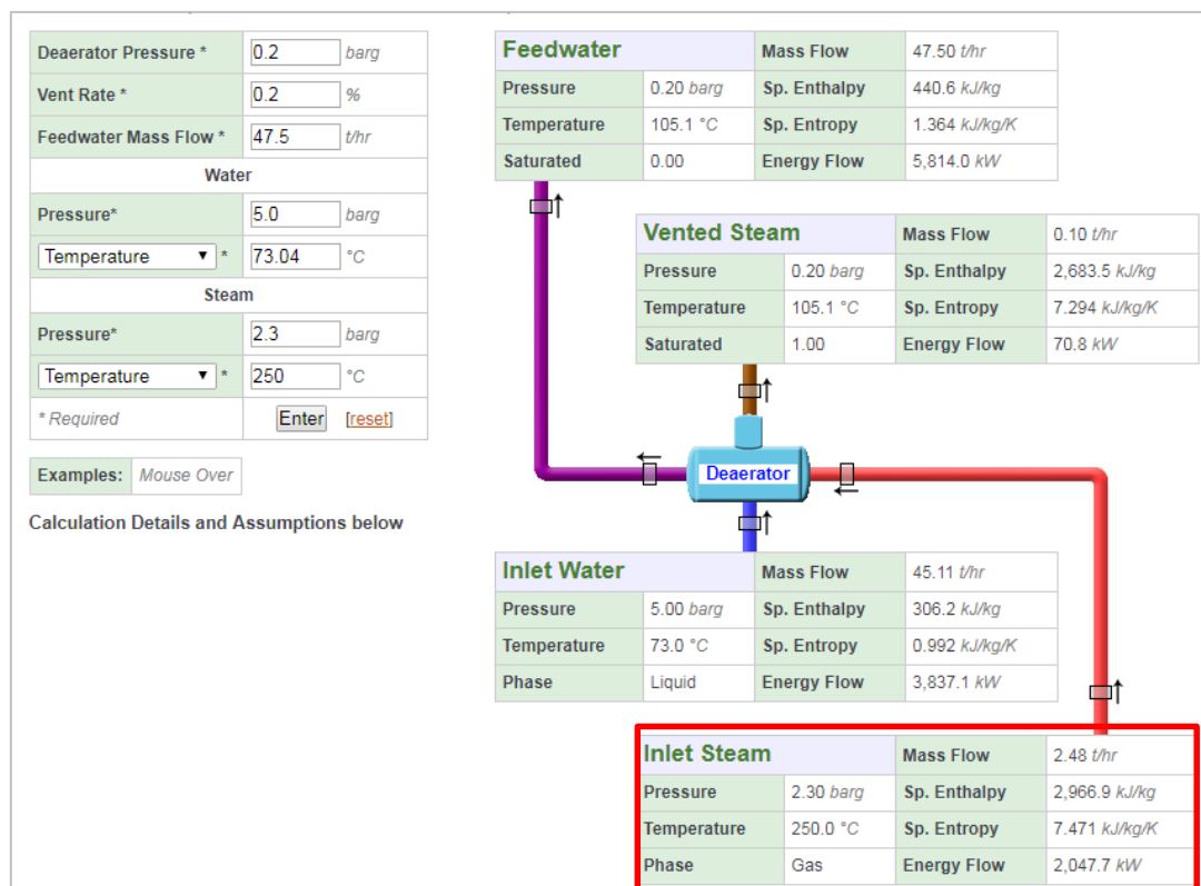
รูปที่ 6.40 การคำนวณปริมาณไอน้ำออกจาก Extraction turbine กลับมาใช้อุ่นน้ำป้อนดีแอโรเตอร์ (หลังการปรับปรุง)
