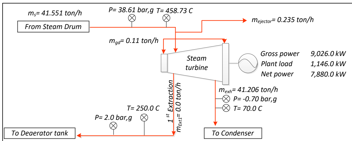
รูปที่ 9.60 ไดอะแกรมการใช้ไอน้ำก่อนการปรับปรุงมาตรการลดความดันไอน้ำขาออกจากกังหันไอน้ำ
