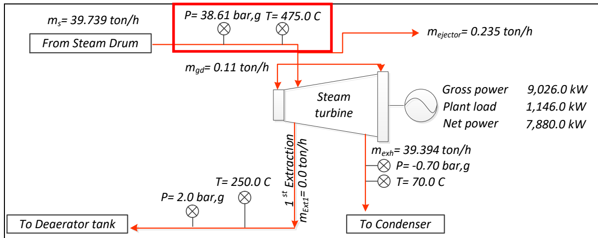
รูปที่ 9.64 ไดอะแกรมการใช้ไอน้ำมามาตรการเพิ่มอุณหภูมิไอน้ำด้วยการลดปริมาณ การสเปรย์น้ำที่ตีซูเปอร์ฮีเตอร์
