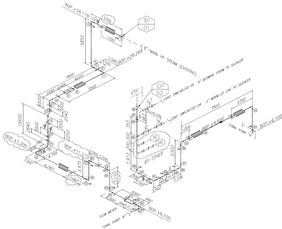
รูปที่ 10.5 Main Steam Piping Line และ Pipe Support
