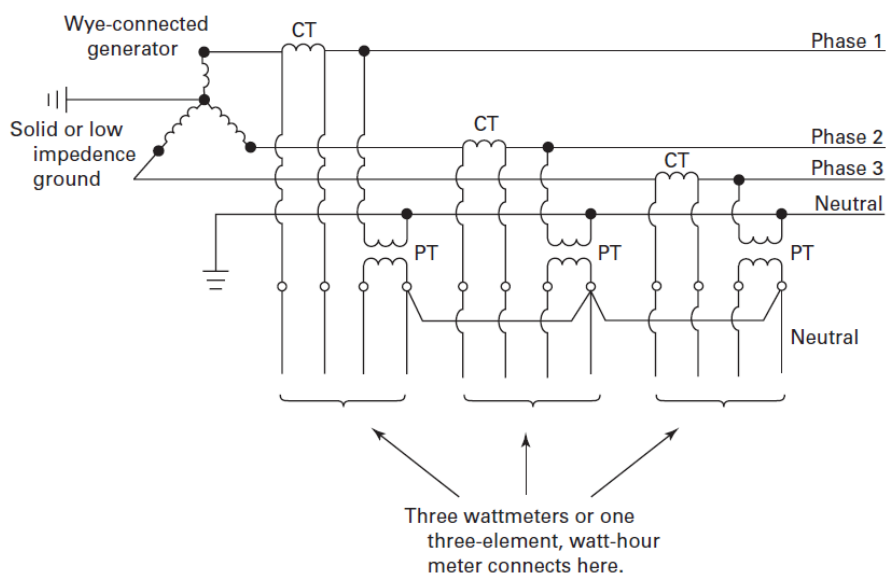
รูปที่ 6.11 การวัดกำลังไฟฟ้า แบบ Four-Wire System
