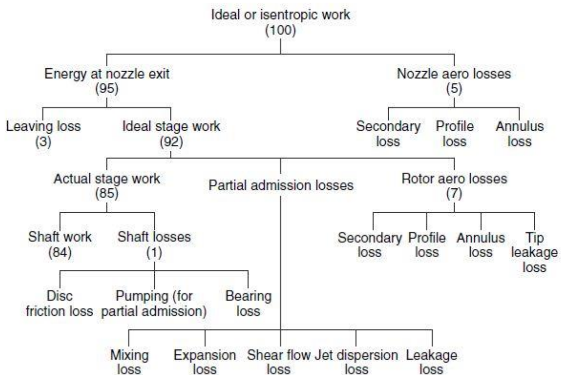
รูปที่ 6.16 การประมาณค่าความสูญเสียต่างๆของกังหันไอน้ำ
