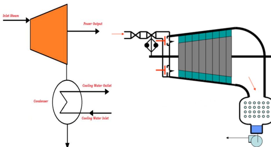
รูปที่ 6.1 แผงผังของ Condensing turbine
