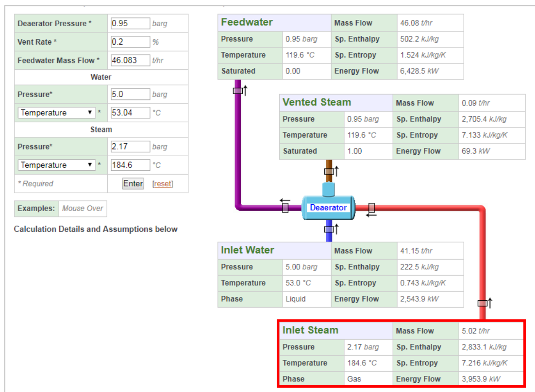
รูปที่ 9.45 การประเมินการใช้ไอน้ำอุ่นน้ำป้อนในถังดีแอโรเตอร์ และปริมาณ Vent out (หลังการปรับลดไอน้ำปล่อยทิ้งที่ Vent valve)
