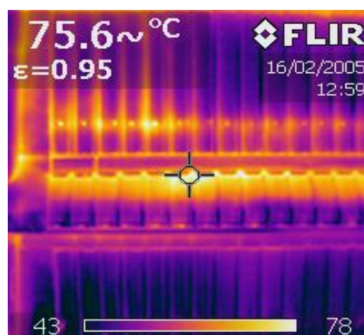
(ง) ภาพถ่ายความร้อนผนังด้านหน้าหม้อน้ำ
