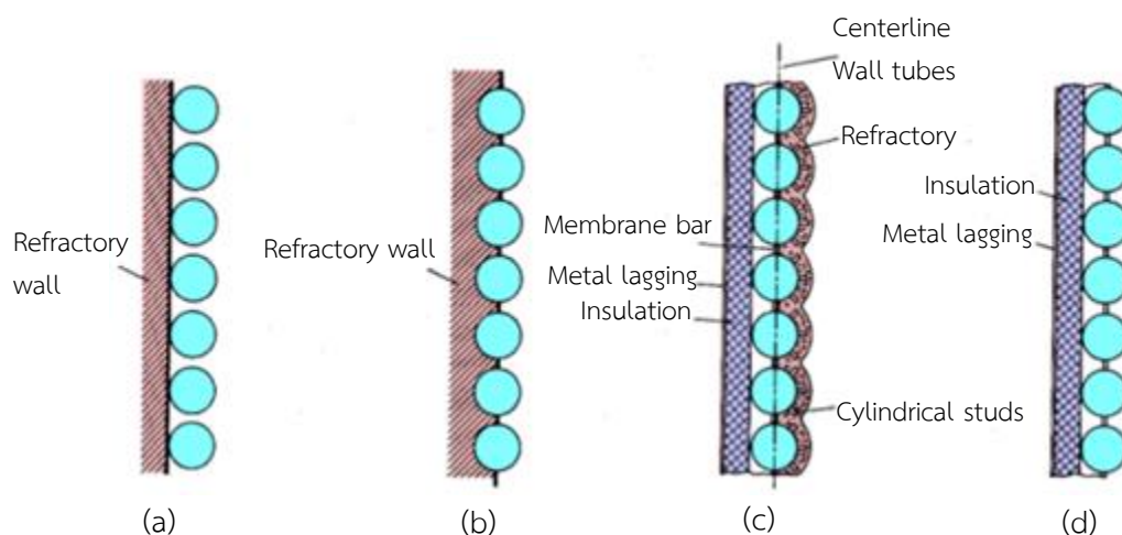
รูปที่ 4.2 เปลือกหม้อน้ำที่เป็นท่อน้ำ
