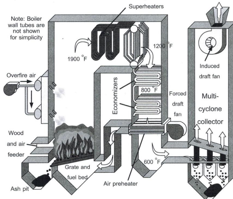
รูปที่ 3.16 เครื่องกำเนิดไอน้ำที่มีระบบมลติไซโคลน
