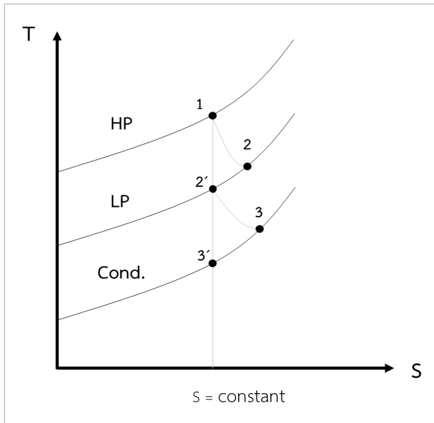
รูปที่ 9.19 เกล็ดการหาประสิทธิภาพไอเซนโทรปิกของกังหันไอน้ำ
