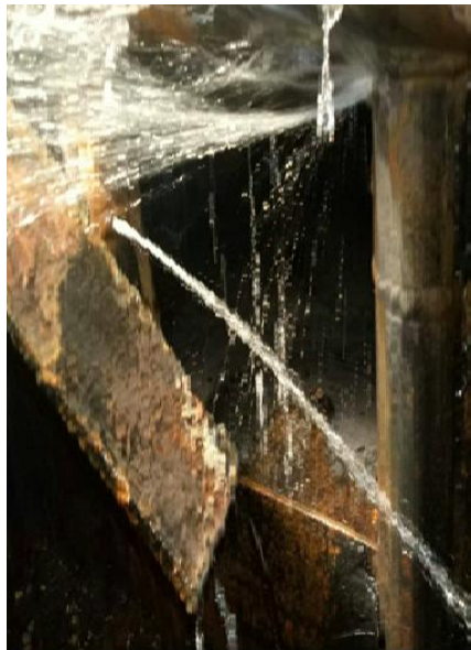
รูปที่ 10.3 Boiler Tube Leak ที่แนวเชื่อมต่อ Back Water Wall Tube กับ Upper Header
