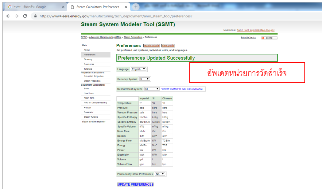
รูปที่ 6.21 ขั้นตอนการเปลี่ยนหน่วยการวัดในโปรแกรม SSMT
