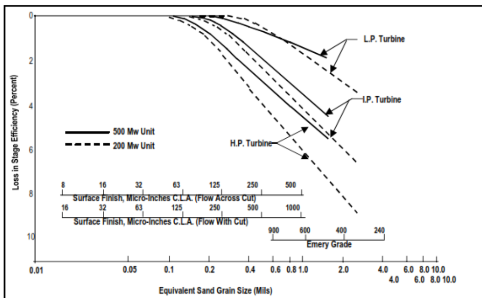
รูปที่ 6.14 ผลกระทบของความเรียบผิวที่มีต่อประสิทธิภาพกังหันไอน้ำ
