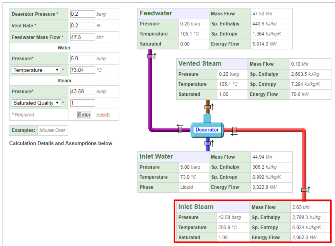
รูปที่ 6.37 การคำนวณปริมาณไอน้ำจากตรัมบนที่ใช้ไอน้ำในดีแอร์เรเตอร์ (ก่อนการปรับปรุง)
