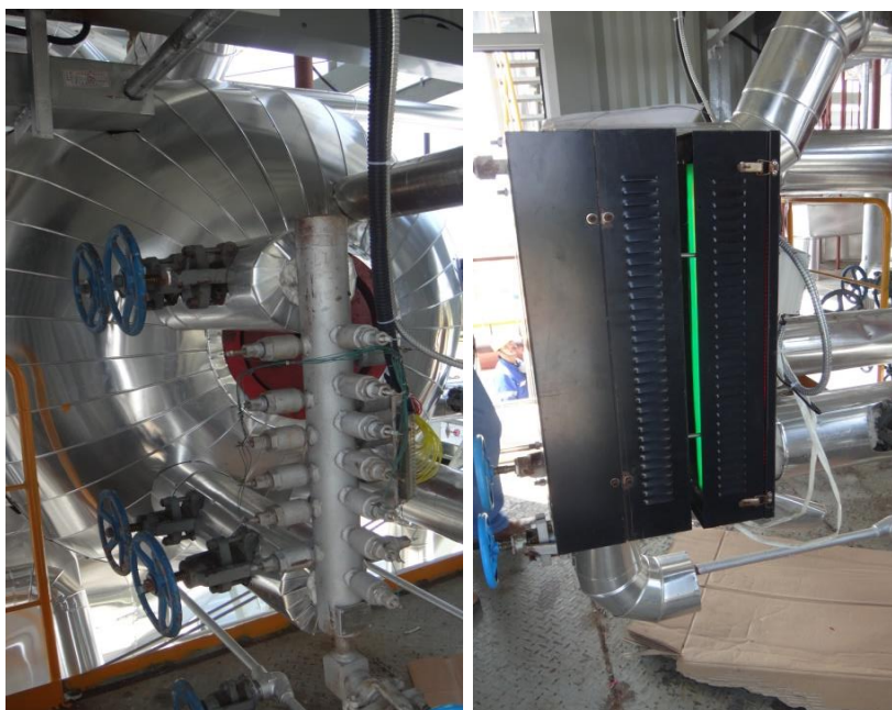
รูปที่ 10.16 สภาพชุด Sigh Glass และ Electrode ช่วงติดตั้ง Plant ใหม่
