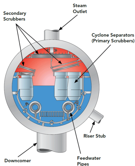
รูปที่ 4.5 (ค) การแยกไอน้ำโดยวิธีต่างๆ ในถังพักไอน้ำ แบบแรงหนีศูนย์กลาง (Centrifugal) [ที่มา : https://www.babcock.com/products/radiant-boiler ]
