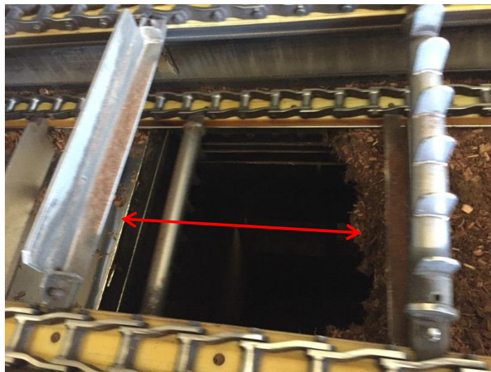
รูปที่ 9.58 Fuel hopper chute
