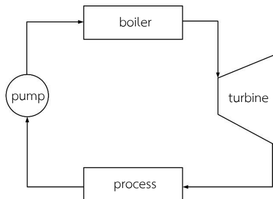
รูปที่ 2.11 ระบบผลิตพลังงานร่วมที่ใช้เครื่องกังหันไอน้ำแบบแรงดันย้อนกลับ
