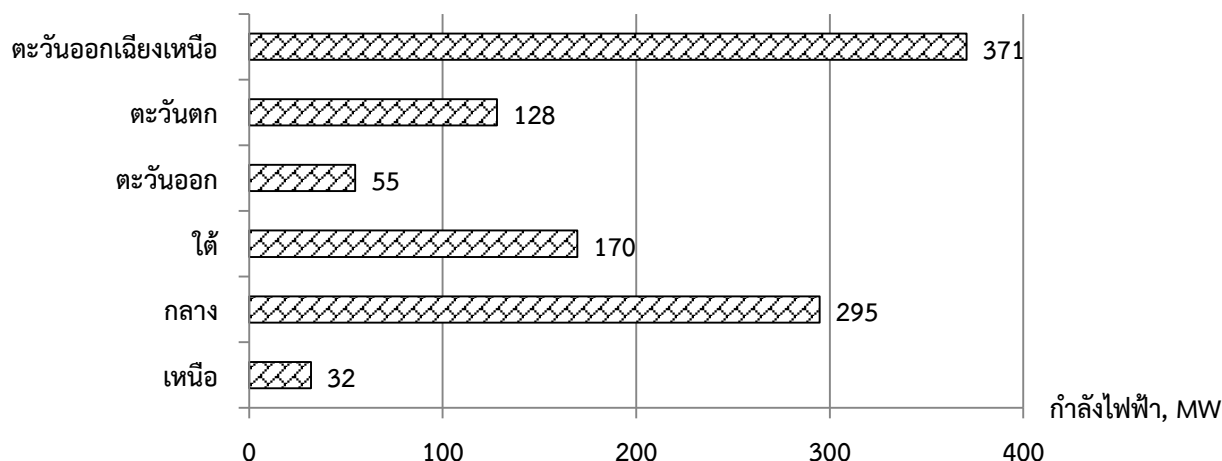
รูปที่ 1.7 กำลังการผลิตไฟฟ้าของโรงไฟฟ้าชีวมวลขนาดเล็กมากในแต่ละภูมิภาค (170 โรงไฟฟ้า)
