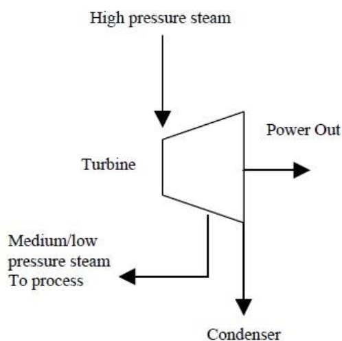
รูปที่ 6.3 แผงผังของ Extraction turbine
