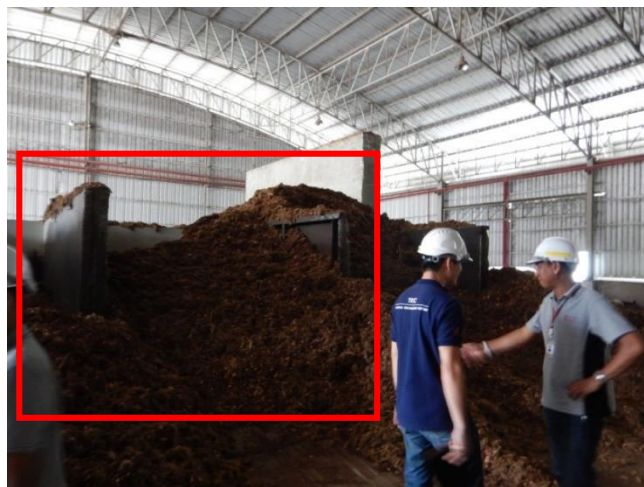
รูปที่ 2.40 บล็อกให้รถตักดันเชื้อเพลิงเข้าถาดลำเลียง (Moving for fuel)
