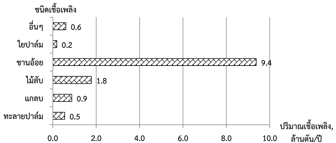
รูปที่ 1.13 ปริมาณการใช้เชื้อเพลิงชนิดต่างๆ ในโรงไฟฟ้าชีวมวลขนาดเล็กมาก (ข้อมูลจากแบบสอบถาม 70 โรงไฟฟ้า)
