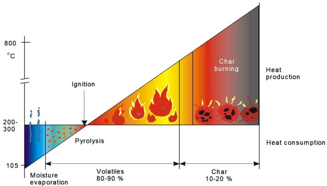
รูปที่ 2.65 การเผาไหม้เชื้อเพลิงชีวมวล
