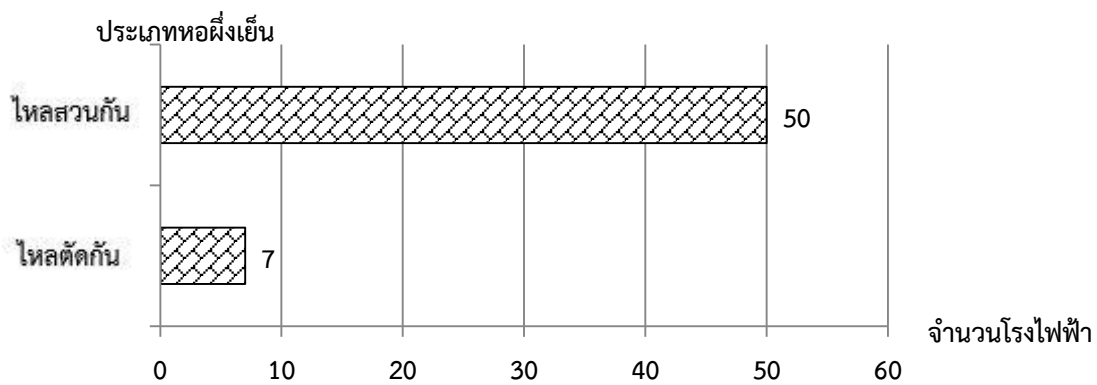
รูปที่ 1.26 ประเภทของห่อฝังเย็นที่ใช้ในโรงไฟฟ้าชีวมวลขนาดเล็กมาก (ข้อมูลจากแบบสอบถาม 70 โรงไฟฟ้า)
