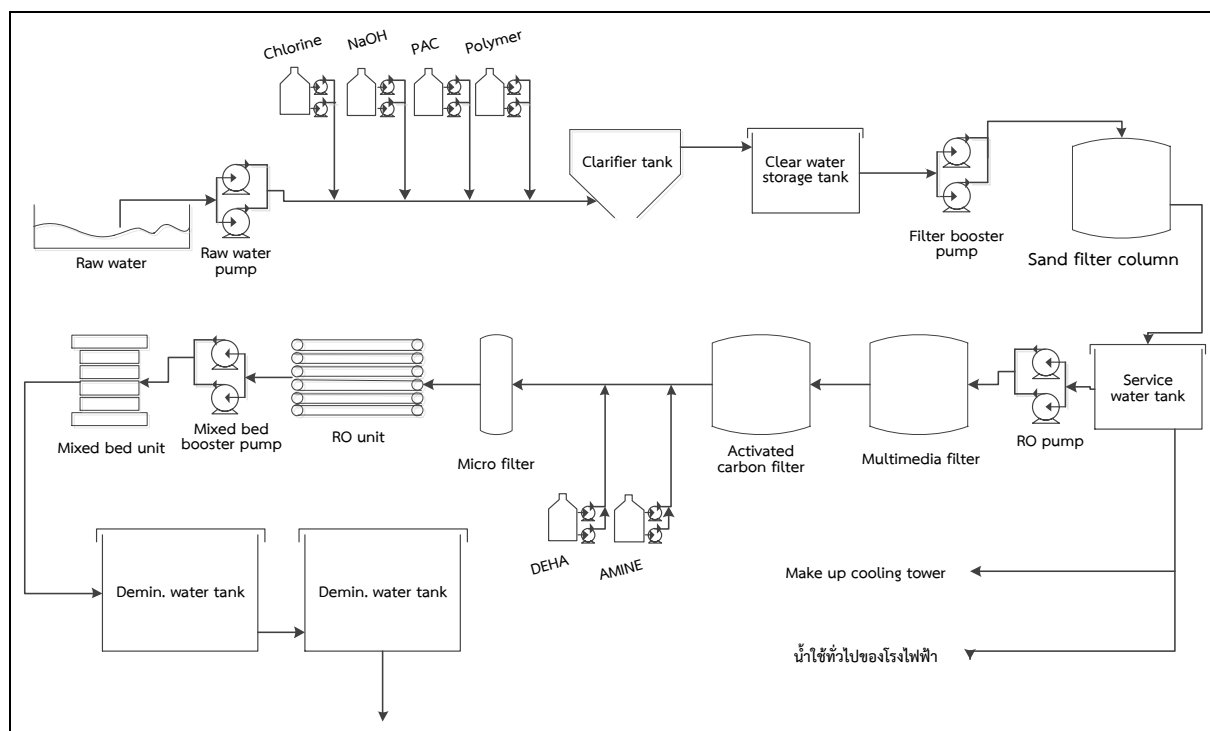
รูปที่ 2.15 แผนผังระบบปรับปรุงคุณภาพน้ำ
