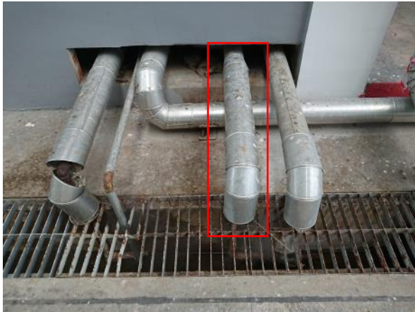
(ก) Steam trap รั่วสติก่อนเข้าถังหาน้ำ
