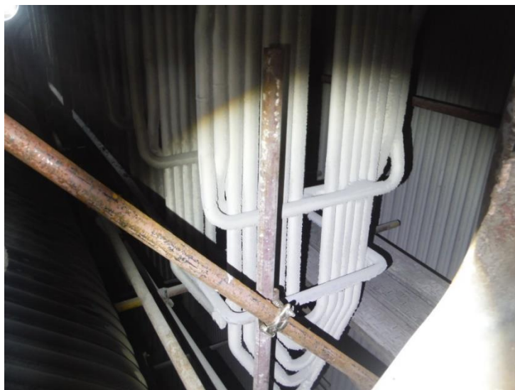
รูปที่ 10.63 สภาพท่อ Platen Superheater Tube
