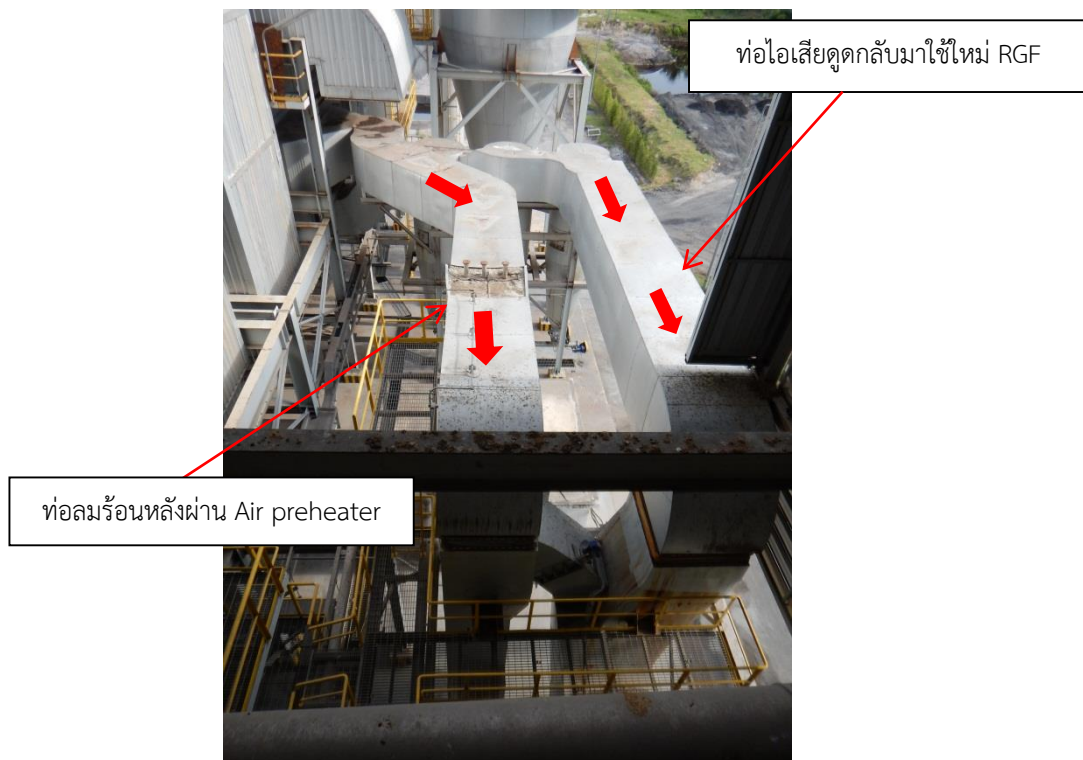
รูปที่ 2.55 ท่อลมร้อนหลังผ่าน Air preheater ด้านซ้าย และท่อดูดไอเสียกลับมาใช้เผาไหม้ซ้ำ RGF (Recirculation gas fan)
