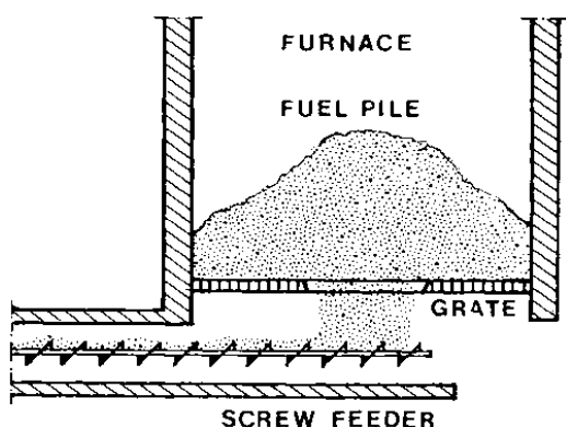
รูปที่ 3.4 การป้อนเชื้อเพลิงจากใต้ถ่างแนวนอน (Underfeed stoker, horizontal)
