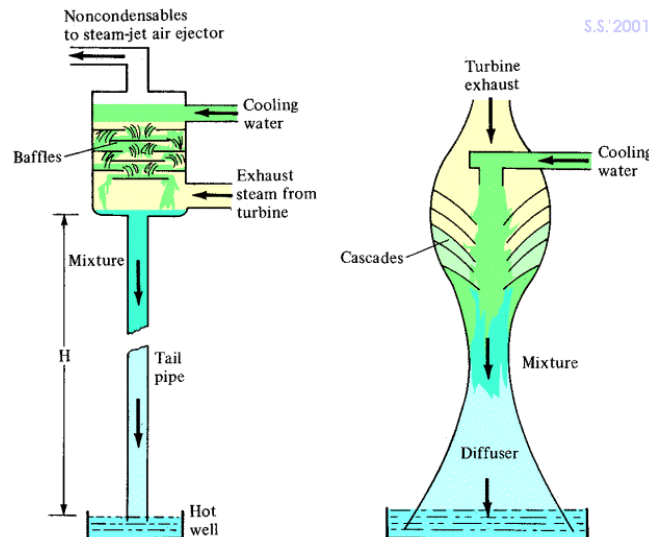
รูปที่ 1.22 Barometric condenser (ซ้าย) และ Jet condenser (ขวา)
