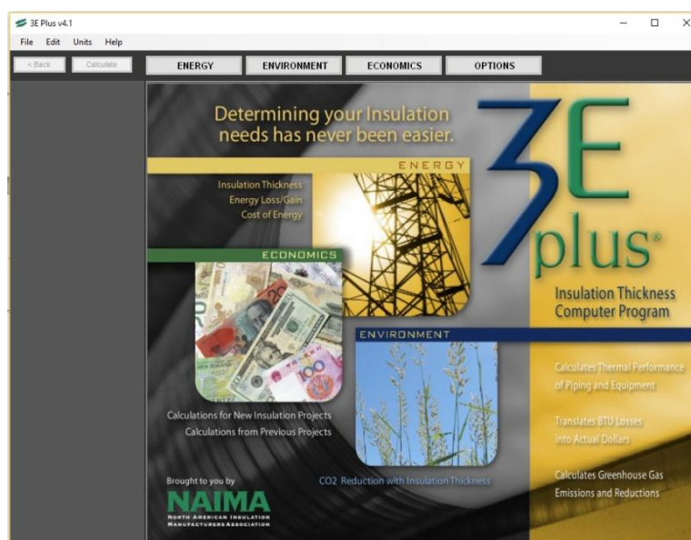
รูปที่ 9.8 โปรแกรม 3E PLUS สำหรับใช้ประเมินการสูญเสียความร้อน
