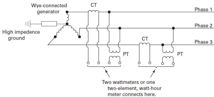
รูปที่ 6.9 การวัดกำลังไฟฟ้า แบบ Three-Wire System (Wye)
