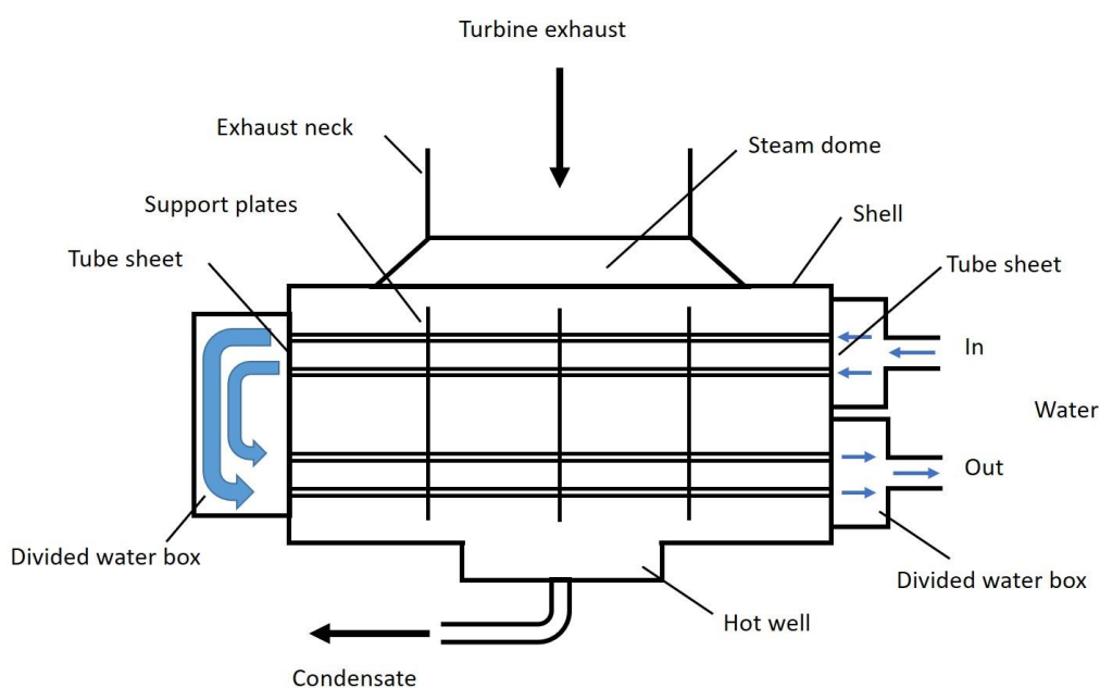
รูปที่ 7.5 แผนภาพของเครื่องควบแน่นแบบผิวสัมผัสไหล 2 ทาง
