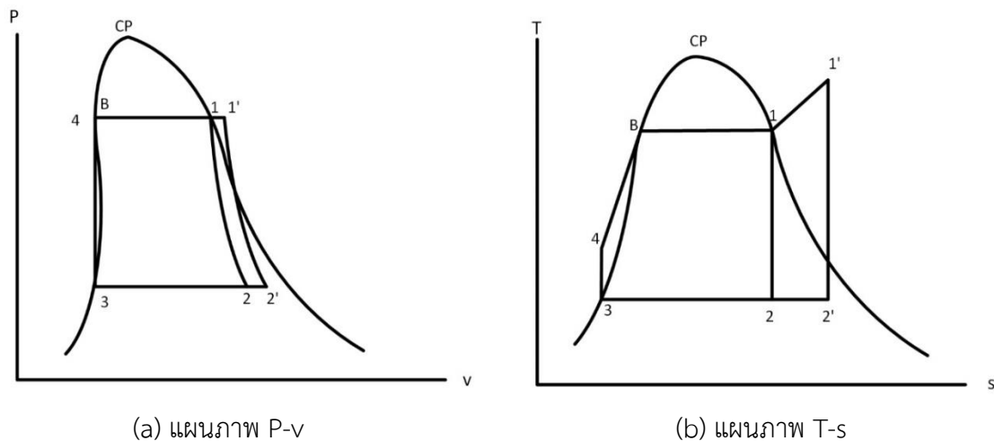
รูปที่ 2.3 แผนภาพ P-v และ T-s ของวัฏจักรแรงคินอย่างง่าย
