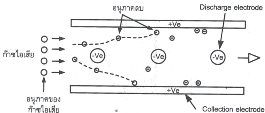
รูปที่ 3.18 หลักการทำงานของเครื่องดักฝุ่นแบบไฟฟ้าสถิต (ESP)
