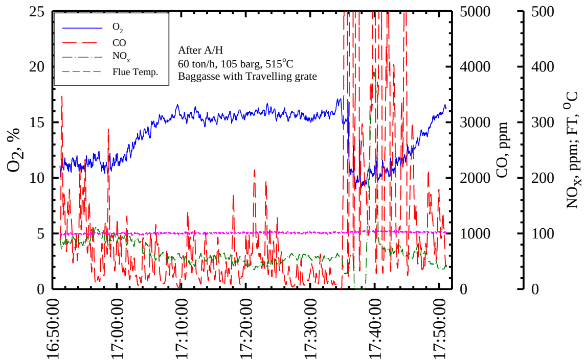
รูปที่ 4.16 ผลการตรวจวัดก๊าซไอเสียของหม้อน้ำโรงไฟฟ้าหลังออก A/H
