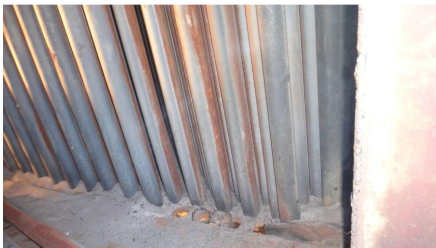
รูปที่ 10.70 ท่อ Air Preheater Tube ที่บาง ต้องทำการตัดเปลี่ยน
