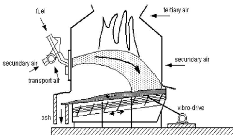
รูปที่ 3.6 ชุดตะกุกหรือหว่านกระจายเชื้อเพลิง
