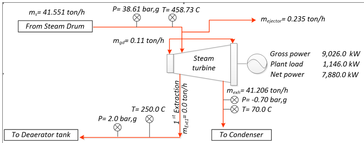
รูปที่ 6.34 ไดอะแกรมการใช้ไอน้ำ ณ วันที่เข้าตรวจวัดกังหันไอน้ำ (Steam turbine)
