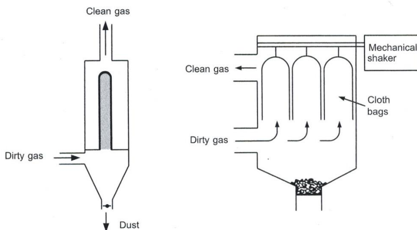
รูปที่ 3.17 ถุงผ้ากรอง (Bag filter)
