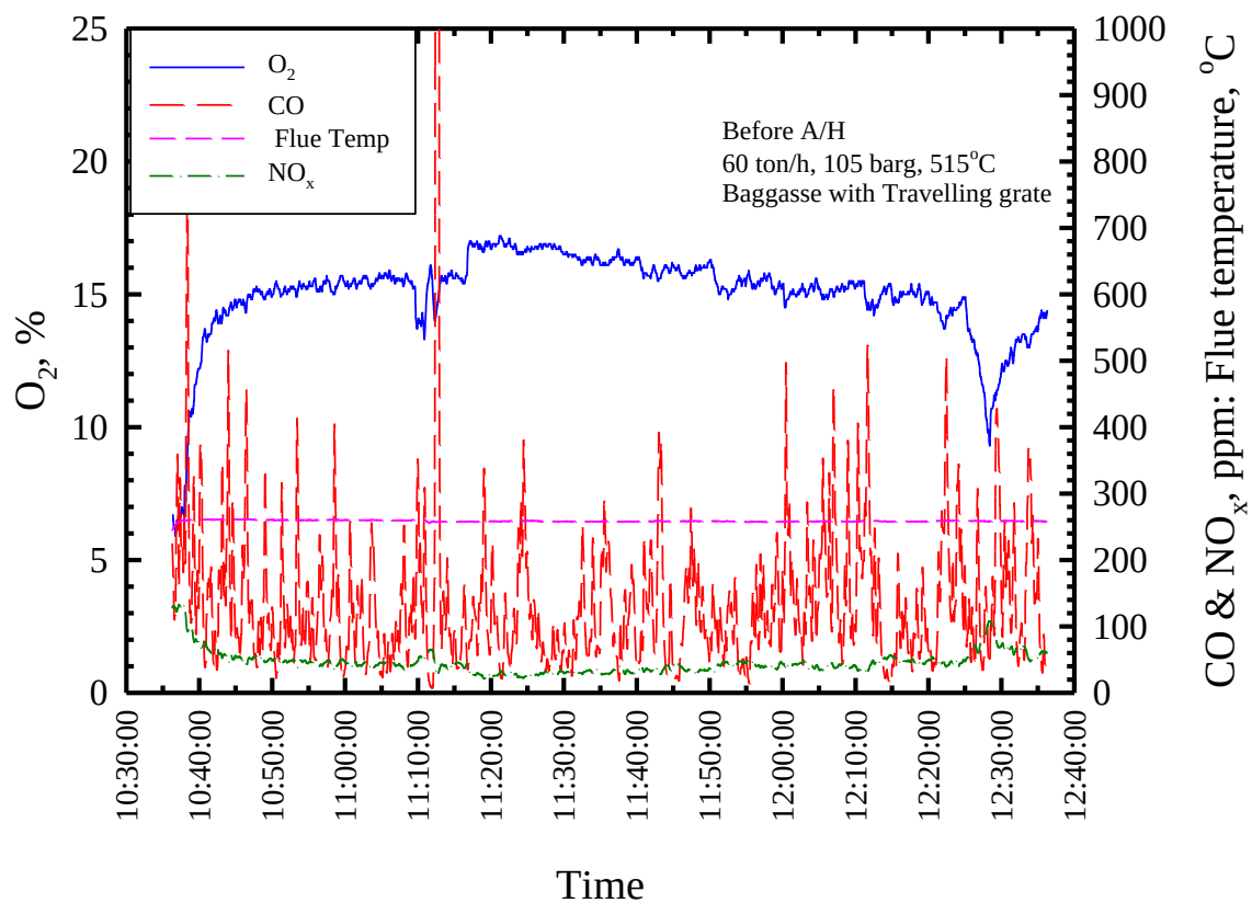
รูปที่ 4.17 ผลการตรวจวัดก๊าซไอเสียของหม้อน้ำโรงไฟฟ้าก่อนเข้า A/H
