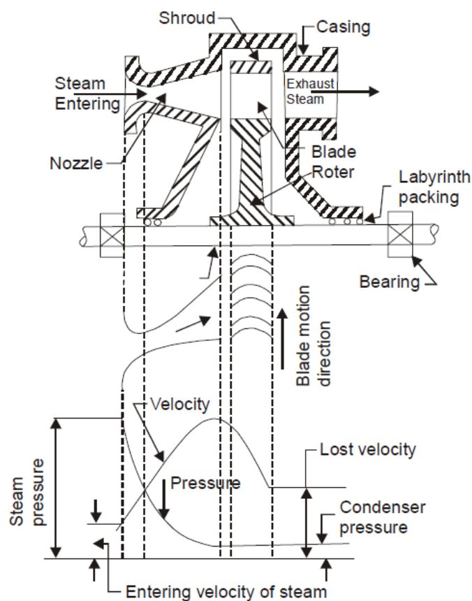
รูปที่ 6.5 แผงผังของ Impulse turbine
