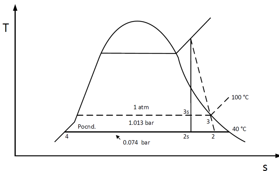
รูปที่ 7.2 การเพิ่มงานต่อหน่วยมวลไอน้ำที่ออกจากกังหันไอน้ำโดยเครื่องควบแน่น
