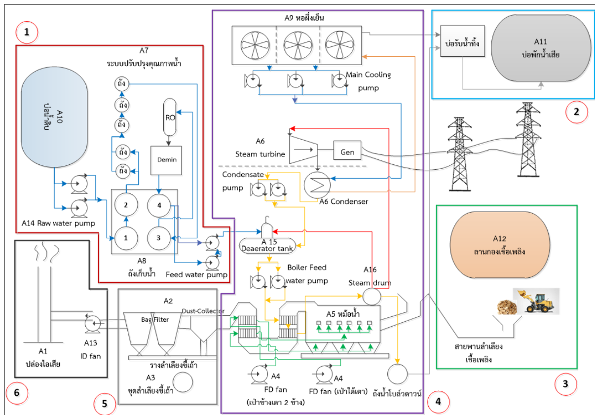
รูปที่ 2.14 ไดอะแกรมระบบต่างๆ ในโรงไฟฟ้า
