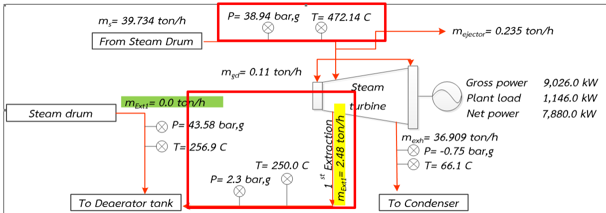
รูปที่ 6.39 แผนผังการใช้ไอน้ำ Steam turbine (หลังการปรับปรุง)
