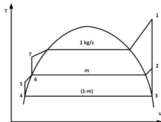
รูปที่ 2.5 วัฏจักรแรงคินที่มีเครื่องอุ่นน้ำป้อนแบบเปิด
