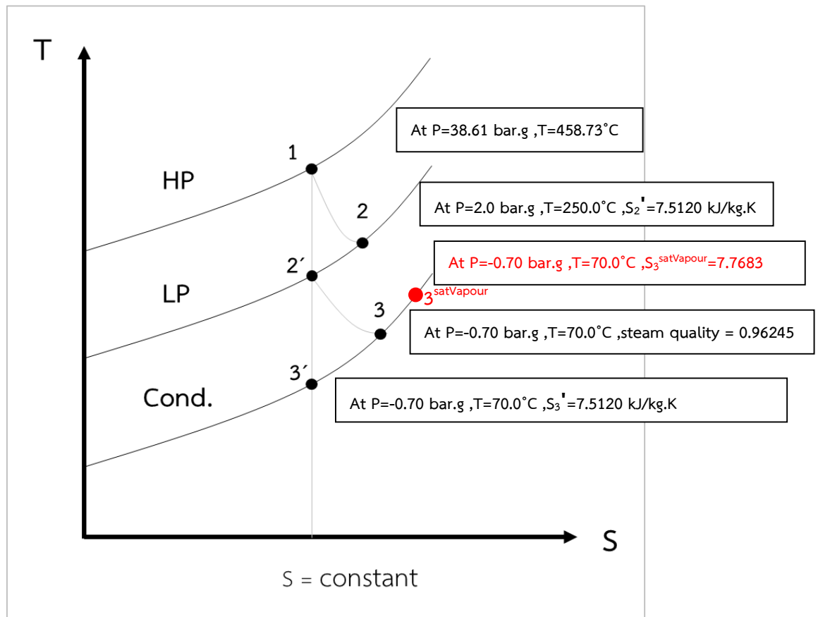
รูปที่ 6.26 กราฟ Isentropic ของ Steam turbine
