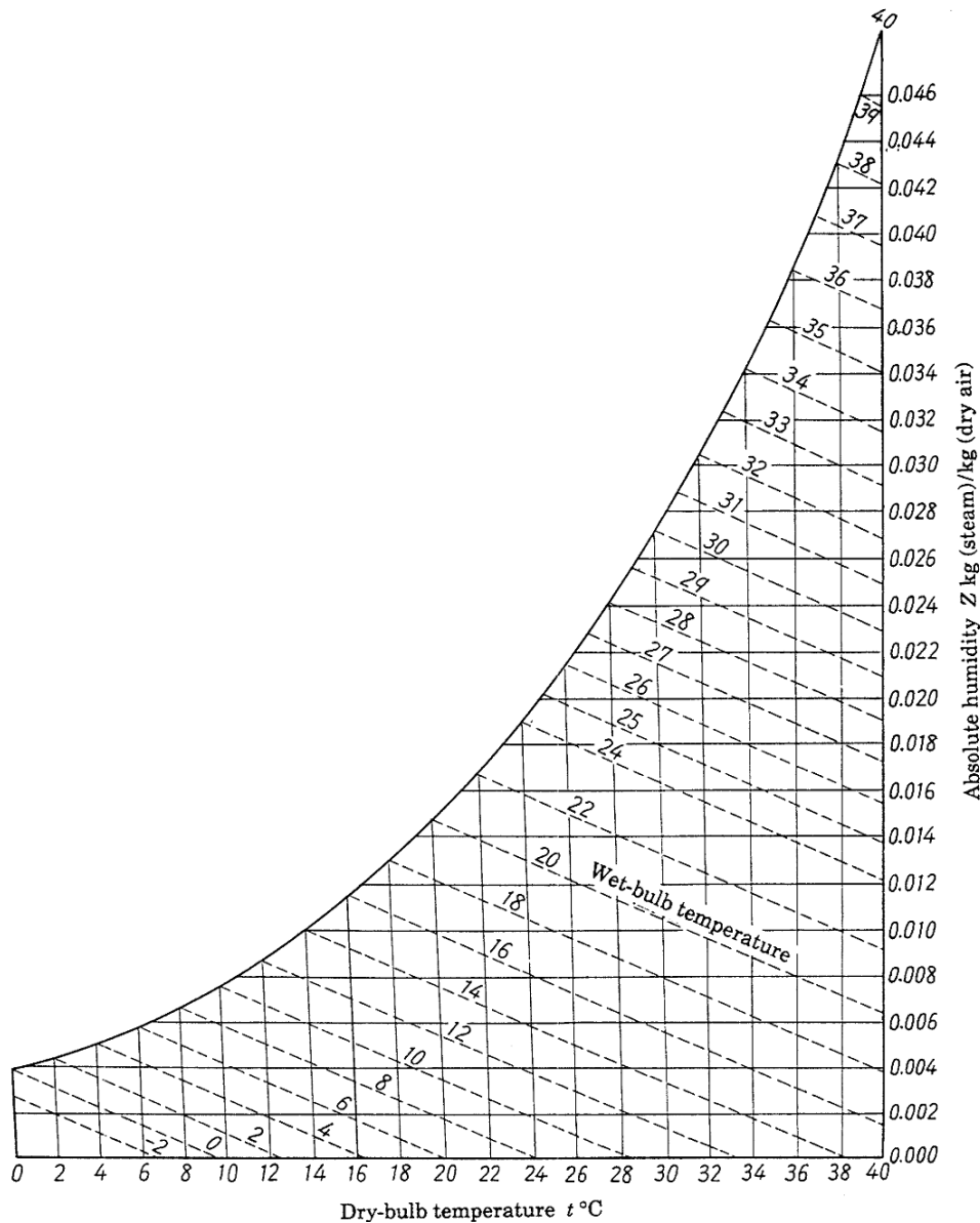
รูปที่ 4.12 ความชื้นสัมบูรณ์ของอากาศ
