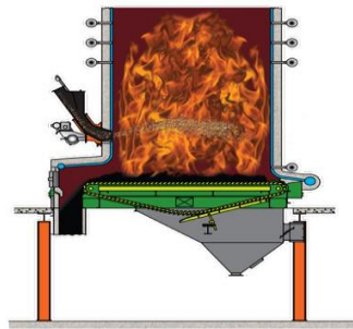
ตะกรับเคลื่อนที่
