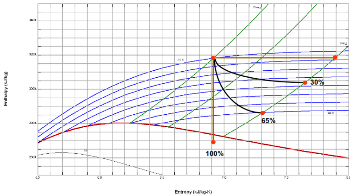
รูปที่ 6.17 Mollier Diagram – Isentropic Turbine Efficiency
