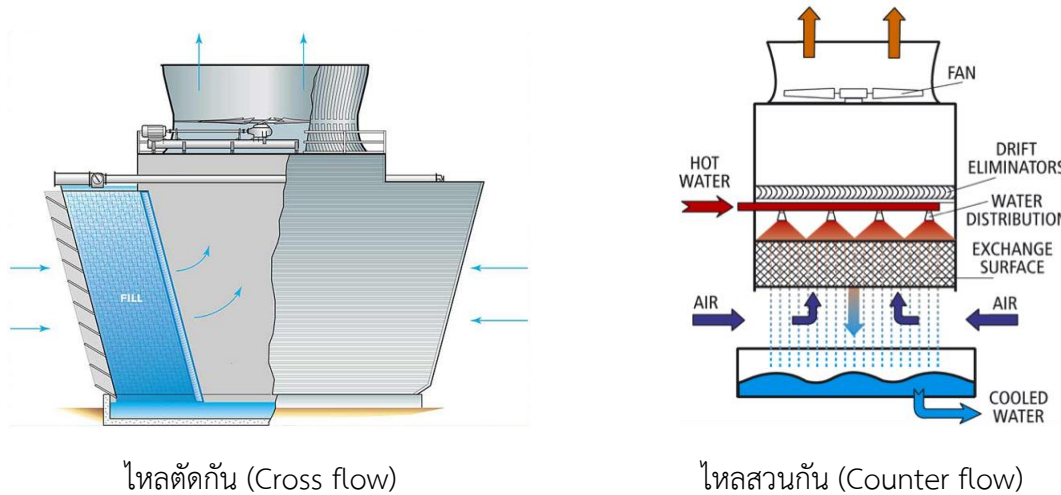
รูปที่ 1.25 ประเภทหอผึ่งเย็นที่ใช้ในโรงไฟฟ้าชีวมวล
