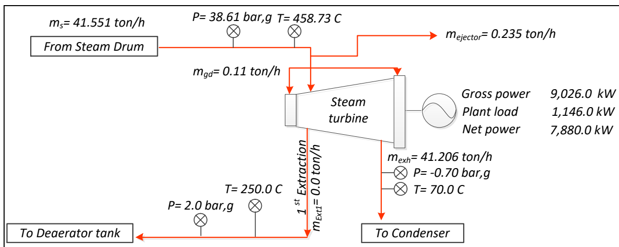
รูปที่ 9.23 ไดอะแกรมการใช้น้ำ ณ วันที่เข้าตรวจวัดกังหันไอน้ำ (Steam turbine)
