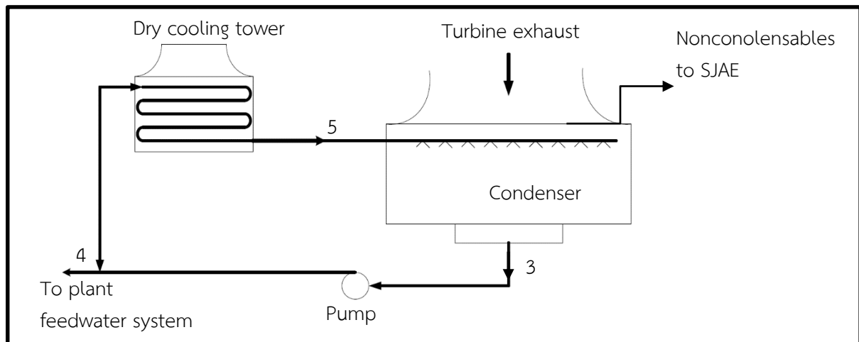
รูปที่ 7.3 เครื่องควบแน่นชนิดแบบสัมผัสโดยตรง
