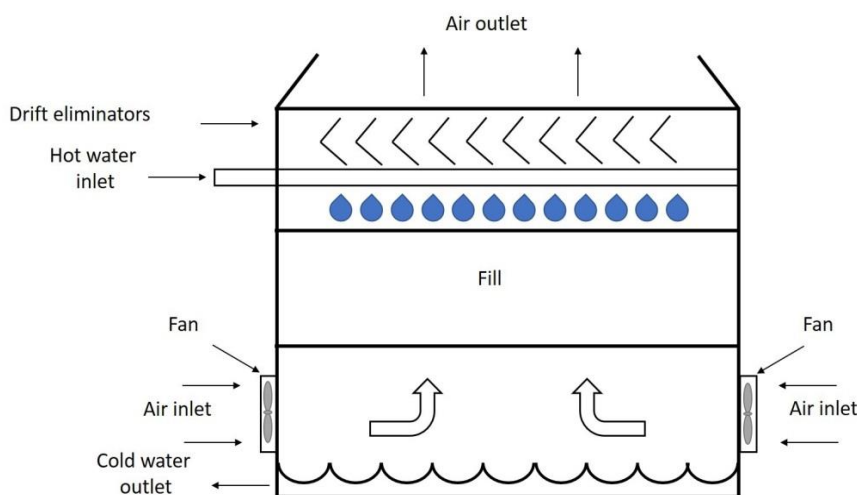
รูปที่ 8.7 หอผึ่งเย็นแบบไหลเวียนแบบเชิงกลแบบเป่าลม (Forced-draft type. FD)
