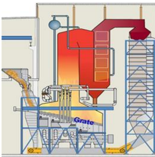
รูปที่ 3.10 ตะกรับไฟเคลื่อนที่กลับไปมา (Reciprocating grate)
