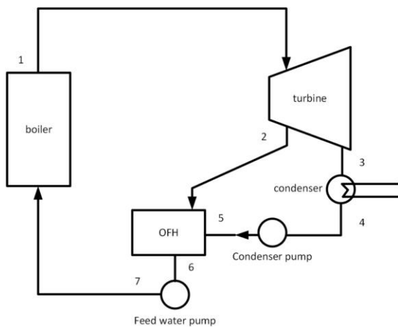
รูปที่ 2.5 วัฏจักรแรงคินที่มีเครื่องอุ่นน้ำป้อนแบบเปิด
