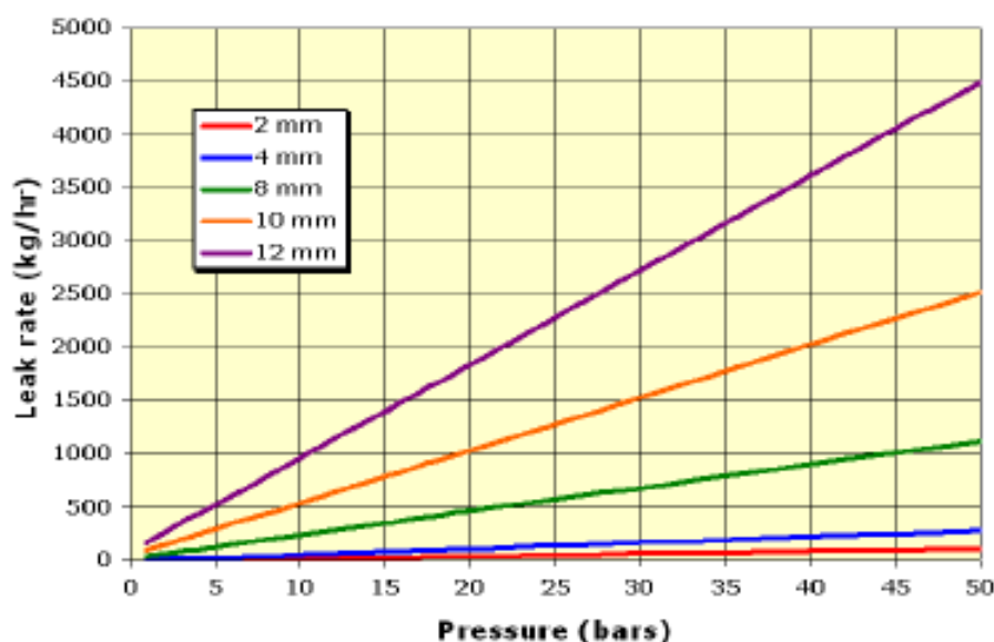
รูปที่ 5.4 ความสัมพันธ์ระหว่างอัตราการรั่วไหลและความดันสัมบูรณ์ที่ขนาดเส้นผ่านศูนย์กลางออร์ฟิศต่างกัน ตามสมการ Napier's choke flow, US DOE SSAT
