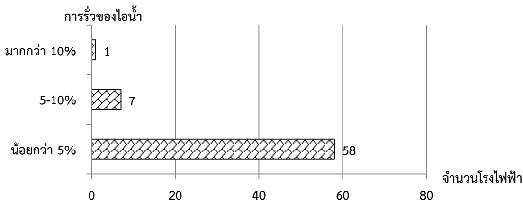
รูปที่ 1.17 สภาพฉนวนในระบบท่อส่งจ่ายไอน้ำของโรงไฟฟ้าชีวมวลขนาดเล็กมาก (ข้อมูลจากแบบสอบถาม 70 โรงไฟฟ้า)
