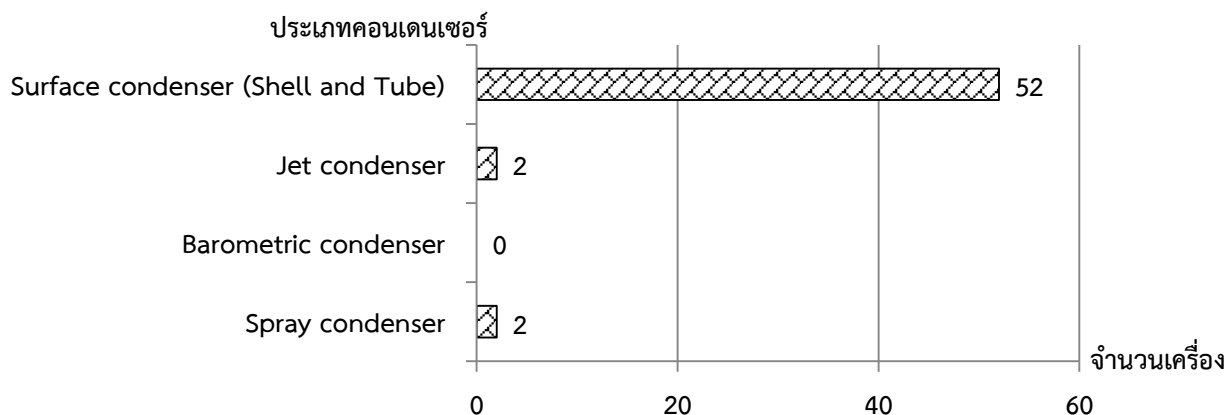
รูปที่ 1.20 ประเภทของคอนเดนเซอร์ที่ใช้ในโรงไฟฟ้าชีวมวลขนาดเล็กมาก (ข้อมูลจากแบบสอบถาม 70 โรงไฟฟ้า)
