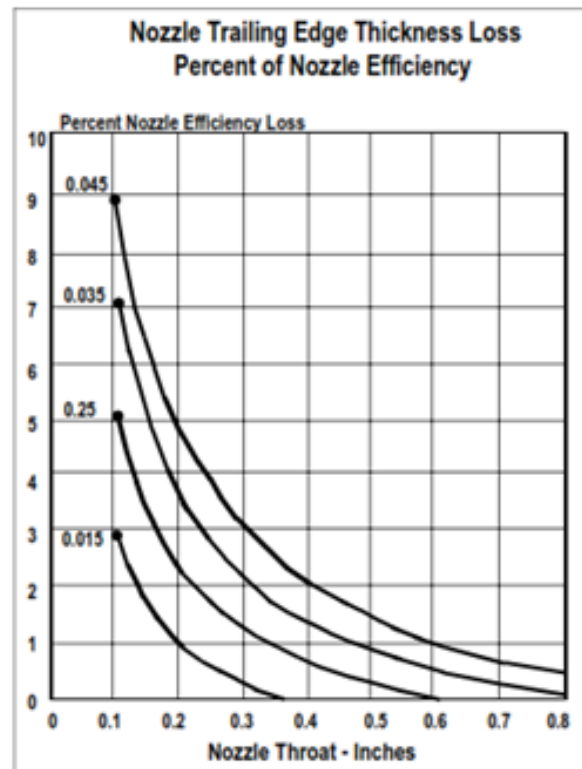
รูปที่ 6.15 ผลกระทบของระยะ Nozzle Throat ที่มีต่อประสิทธิภาพหัวฉีด
