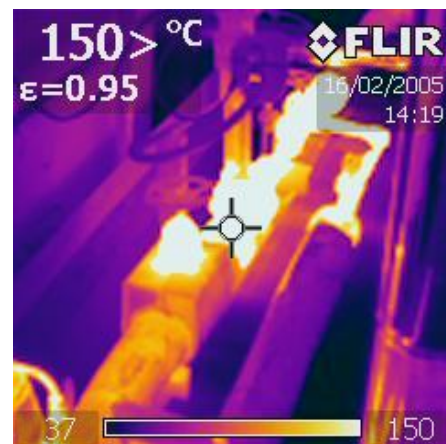
(ง) ภาพถ่ายความร้อน Steam trap รั่วสติก่อนเข้า Deaerator
