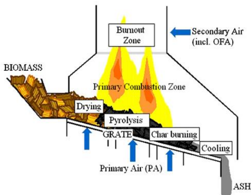
รูปที่ 3.3 การเผาไหม้เชื้อเพลิงชีวมวลในหม้อน้ำ
