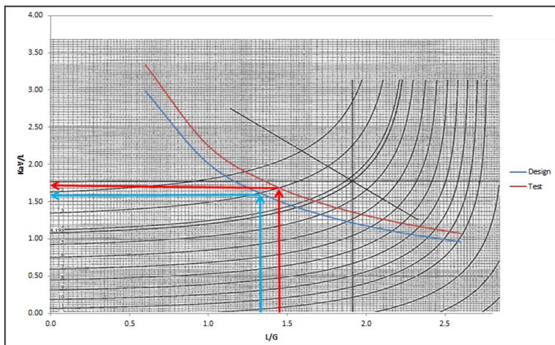
รูปที่ 8.8 กราฟ Tower Demand & Characteristic Curves
