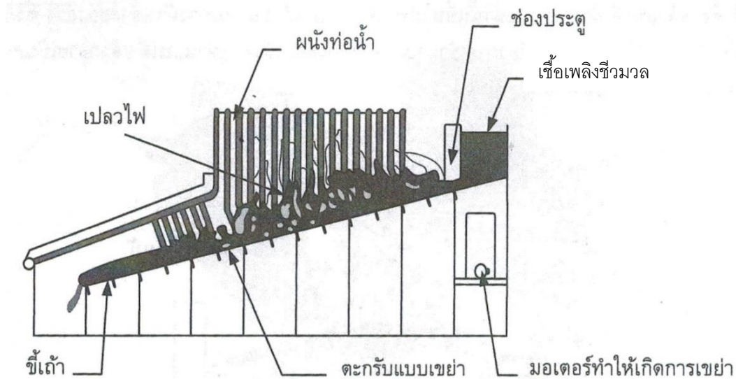
รูปที่ 3.5 ระบบการป้อนเชื้อเพลิงแบบป้อนผ่านช่องประตูที่เป็นตะกรับแบบเขย่า
