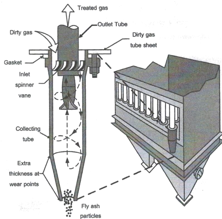
รูปที่ 3.15 มัลติไซโคลน (Multiple cyclones)
