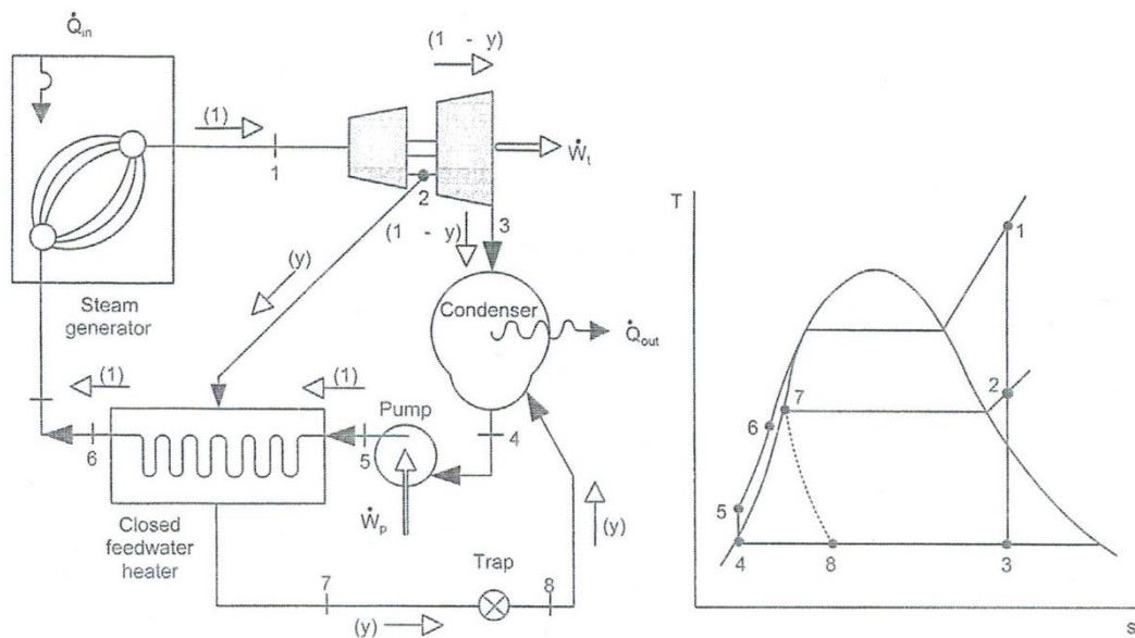
รูปที่ 2.8 แผนภาพของวัฏจักรแรงคินที่มีเครื่องอุ่นน้ำป้อนแบบปิดโดยขับน้ำย้อนกลับ แสดงให้เห็นกับดักไอน้ำ (Steam trap)
