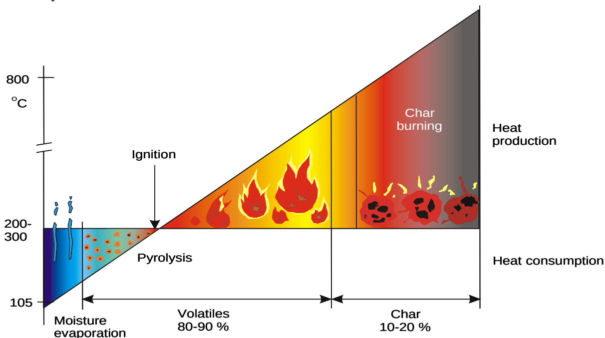
รูปที่ 3.2 กระบวนการเผาไหม้เชื้อเพลิงชีวมวล
