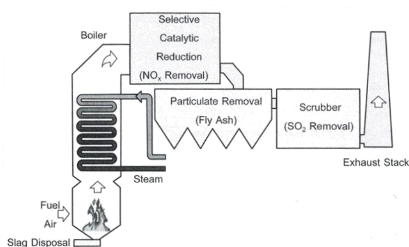
รูปที่ 3.12 ระบบกำจัดมลภาวะทางอากาศของโรงไฟฟ้า
