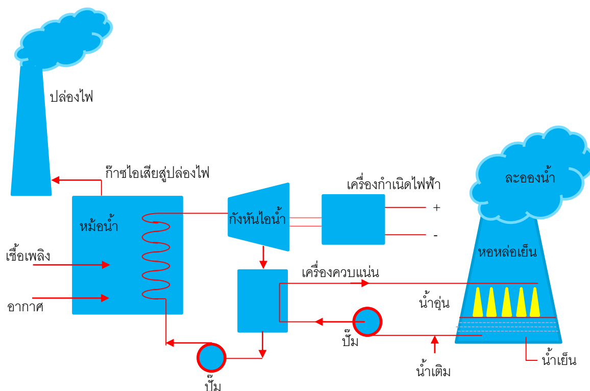
รูปที่ 2.1 ส่วนประกอบของโรงไฟฟ้ากำลังไอน้ำอย่างง่าย
