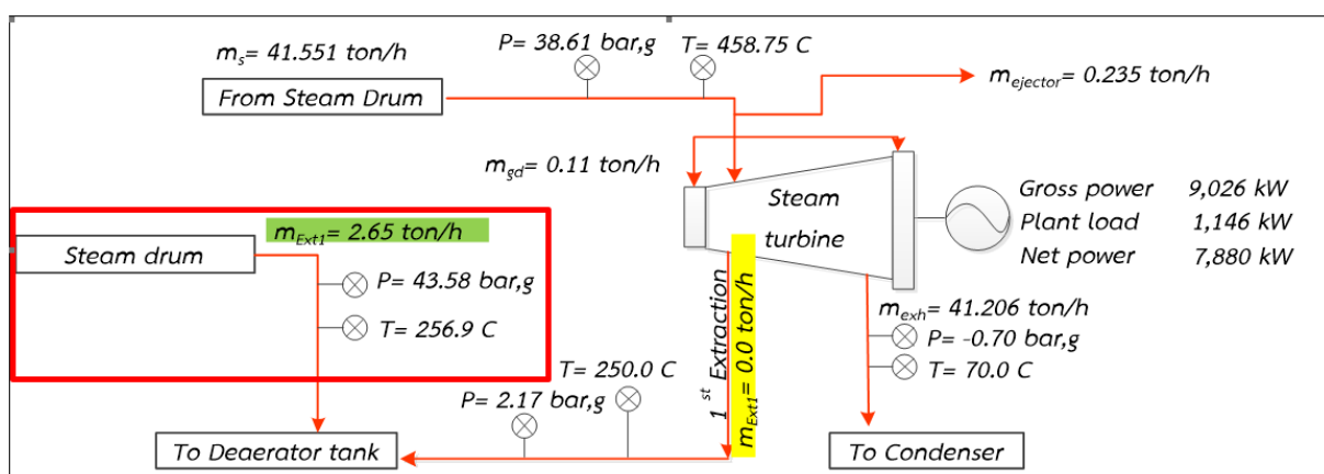
รูปที่ 6.36 แผนผังการใช้น้ำ Steam turbine (ก่อนการปรับปรุง)
