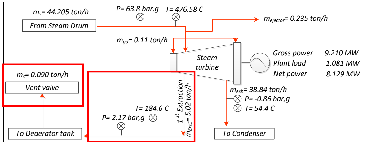
รูปที่ 9.44 ไดอะแกรมการใช้ไอน้ำมามาตรการปรับลดปริมาณไอน้ำใช้ไล่ออกซิเจนในถังดีแอโรเตอร์ (หลังการปรับลดไอน้ำปล่อยทิ้งที่ Vent valve)
