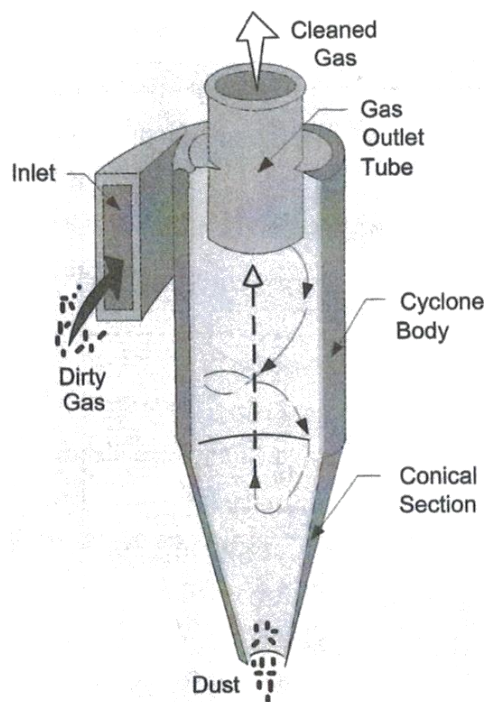
รูปที่ 3.14 ไซโคลน (Cyclone)
