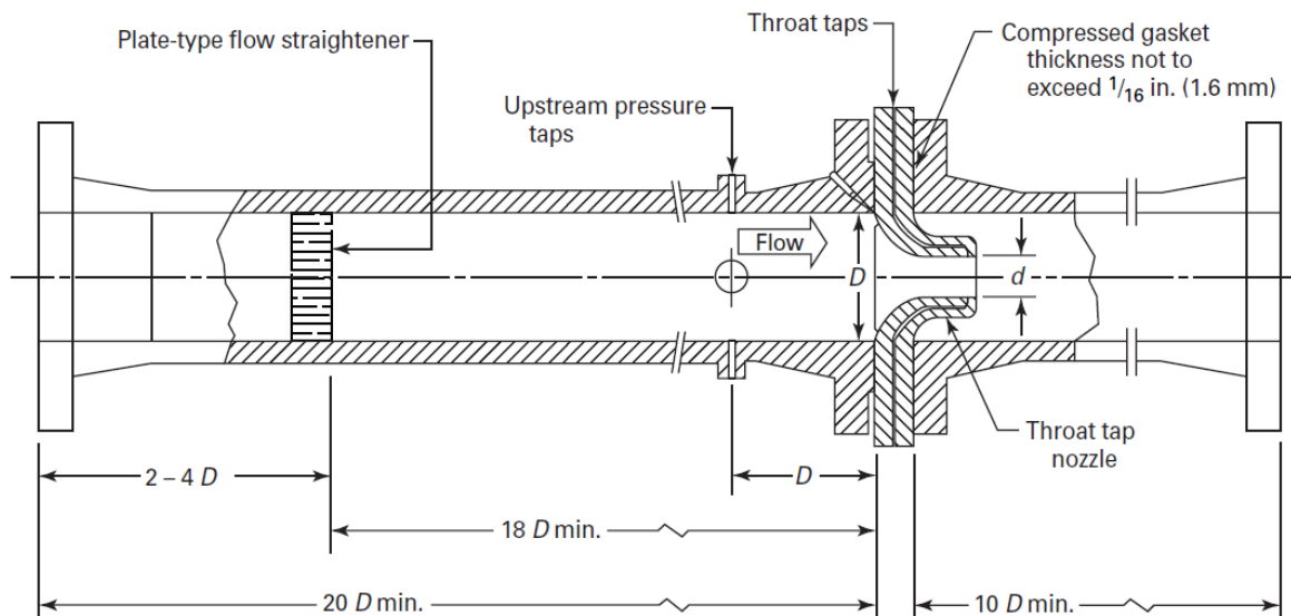
รูปที่ 6.7 การติดตั้งเครื่องวัดอัตราการไหล
