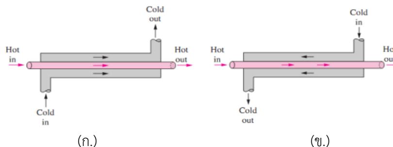
รูปที่ 7.8 หลักการแลกเปลี่ยนความร้อนของเครื่องแลกเปลี่ยนความร้อนแบบ 2 ชั้น
