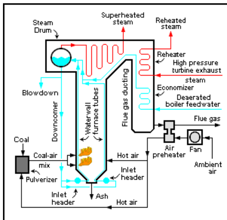
รูปที่ 4.1 ส่วนประกอบของเครื่องกำเนิดไอน้ำสำหรับโรงไฟฟ้า
