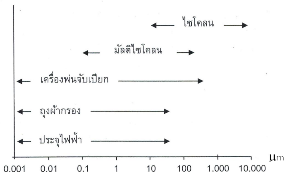
รูปที่ 3.13 ขนาดของฝุ่นเขม่าที่เครื่องจับฝุ่นแต่ละชนิดสามารถจับได้
