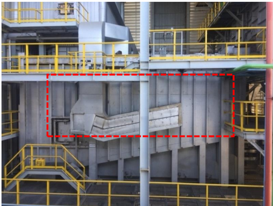
รูปที่ 2.52 หม้อน้ำตะกรับเตาแบบเคลื่อนที่ไป-มา (Reciprocating grate) (ต่อ)
