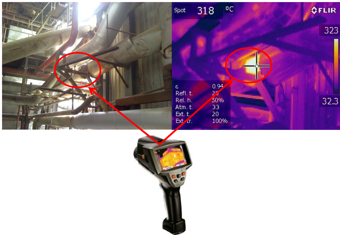
รูปที่ 5.8 ท่อไอน้ำที่ไม่ได้ทำการหุ้มฉนวน
