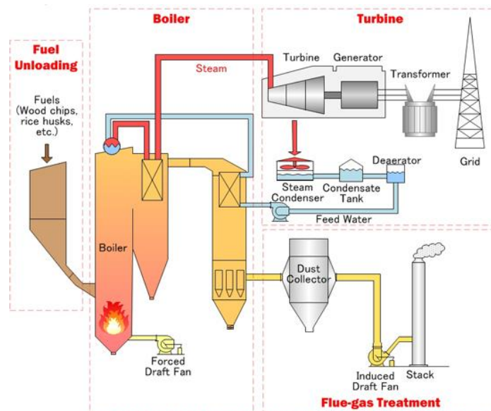
รูปที่ 1.5 แผนผังการทำงานของโรงไฟฟ้าชีวมวล
