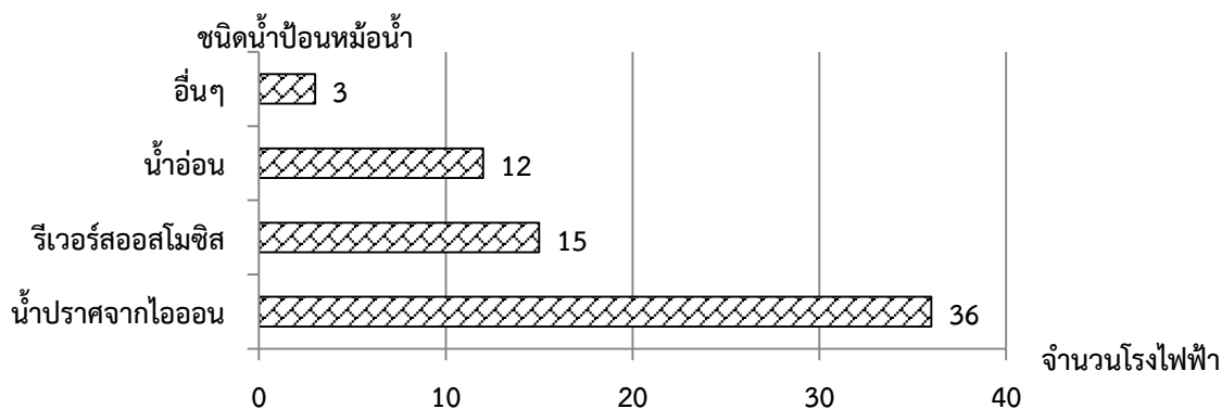
รูปที่ 1.15 ชนิดน้ำป้อนหม้อน้ำโรงไฟฟ้าชีวมวลขนาดเล็กมาก (ข้อมูลจากแบบสอบถาม 70 โรงไฟฟ้า)
