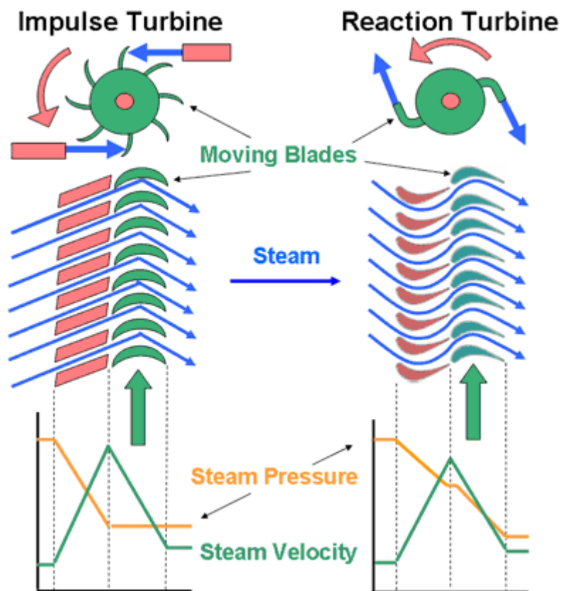
รูปที่ 6.6 แผนผังของการทำงานของ Impulse turbine และ Reaction turbine
