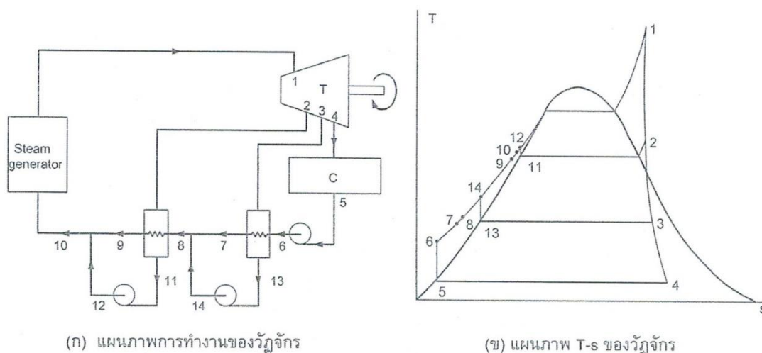
รูปที่ 2.9 วัฏจักรแรงคินไอดงอุดมคติ ติดตั้งเครื่องอุ่นน้ำป้อนแบบปิดโดยใช้ปั๊มขับน้ำไปด้านหน้า
