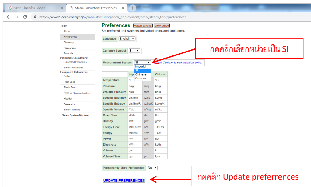
รูปที่ 6.20 ขั้นตอนการเปลี่ยนหน่วยการวัดในโปรแกรม SSMT
