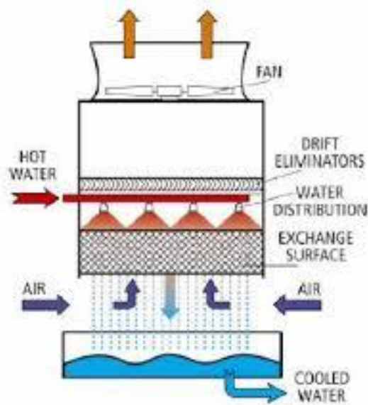
(ข) แผนภาพการทำงาน
