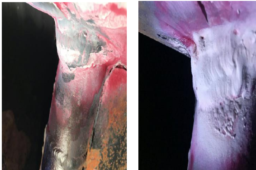
รูปที่ 10.4 การแก้ไข Boiler Tube Leak ที่แนวเชื่อมต่อ Back Water Wall Tube
