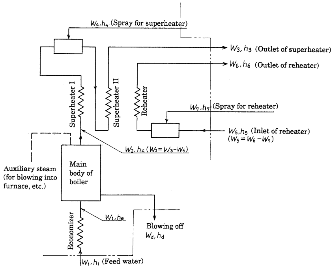
รูปที่ 4.13 ขอบเขตการพิจารณาของการผลิตไอน้ำจากตัวหม้อน้ำหลัก (Main body of boiler) ซุปเปอร์ฮีตเตอร์ (Superheater) รีฮีตเตอร์ (Reheater) และอื่น ๆ
