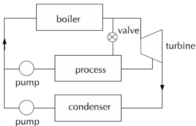
รูปที่ 2.12 ระบบผลิตพลังงานร่วมที่ใช้เครื่องกังหันไอน้ำแบบควบแน่นแยก
