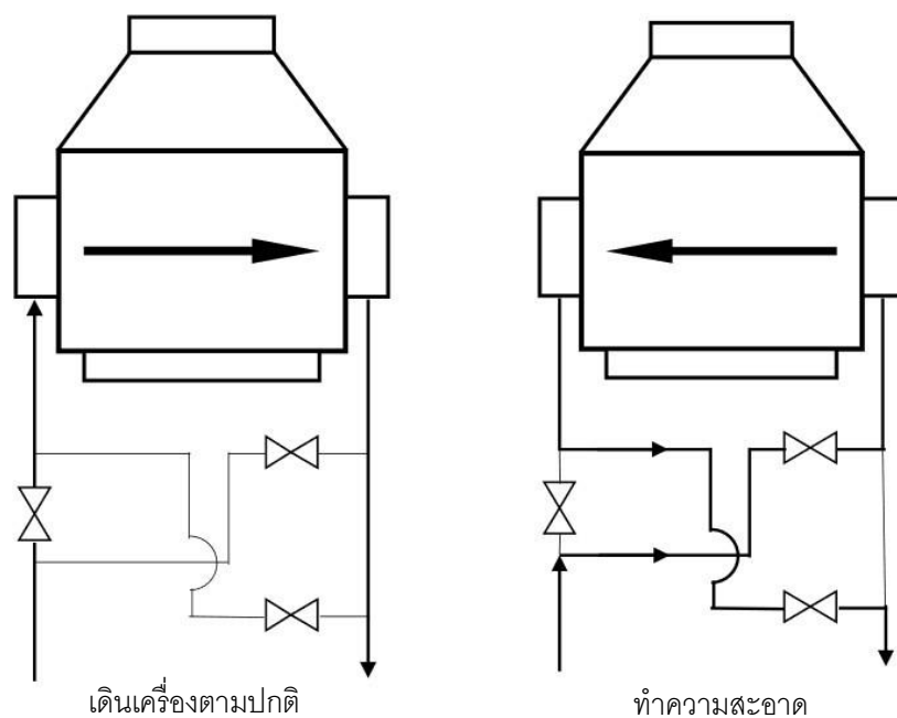
รูปที่ 7.6 วงจรการไหลของเครื่องควบแน่นในสองสภาวะ
