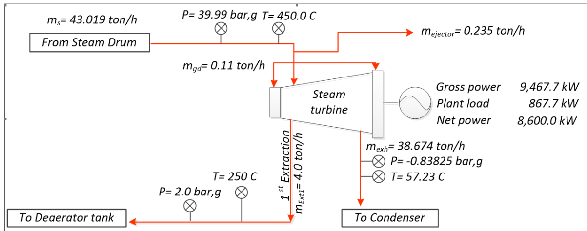
รูปที่ 6.31 ไดอะแกรมการใช้ไอน้ำตามผู้ผลิตออกแบบกังหันไอน้ำ (Steam turbine)
