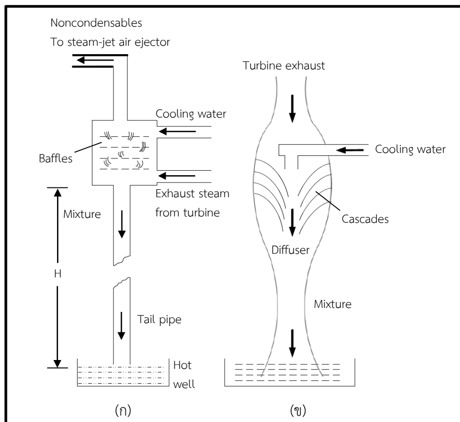
รูปที่ 7.4 (ก) บาร์อมิเตอร์คอนเดนเซอร์ และ (ข) เจ็ตคอนเดนเซอร์
