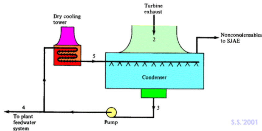
รูปที่ 1.24 Spray condenser
