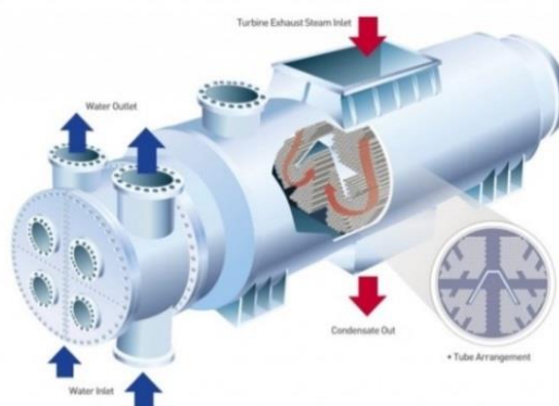
รูปที่ 1.21 Surface condenser
