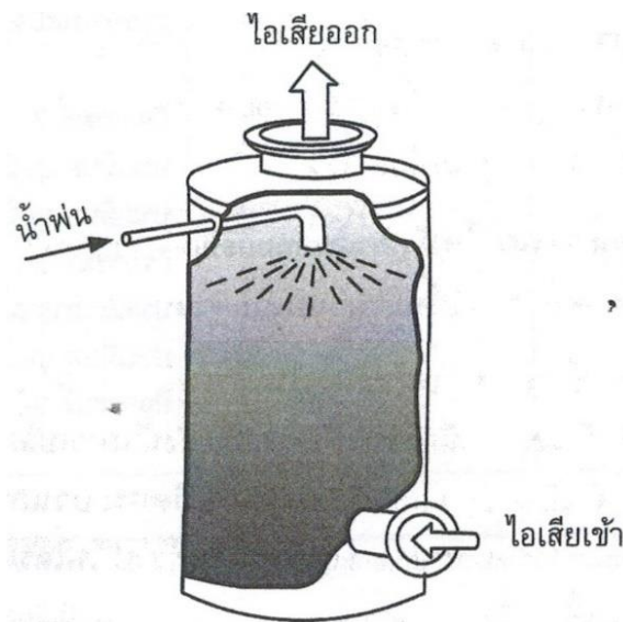
รูปที่ 3.20 เครื่องพ่นจับเปียก (Wet scrubber)
