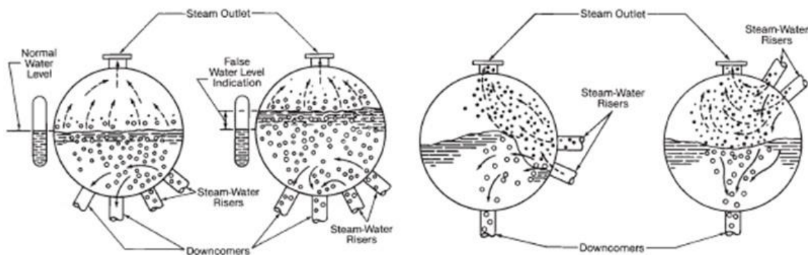
รูปที่ 4.5 (ก) การแยกไอน้ำโดยวิธีต่างๆ ในถังพักไอน้ำ แบบแรงโน้มถ่วง (Gravity)
