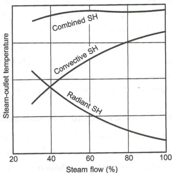
รูปที่ 4.7 การตอบสนองของอุณหภูมิทางออกของการพาความร้อน การแผ่รังสีและผลรวมของทั้งสองในเครื่องดงไอ [Nag, P.K., 2008]
