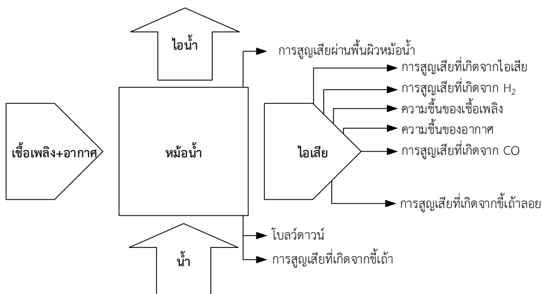
รูปที่ 4.10 แผนผังการประเมินประสิทธิภาพหม้อน้ำด้วยวิธีทางอ้อม
