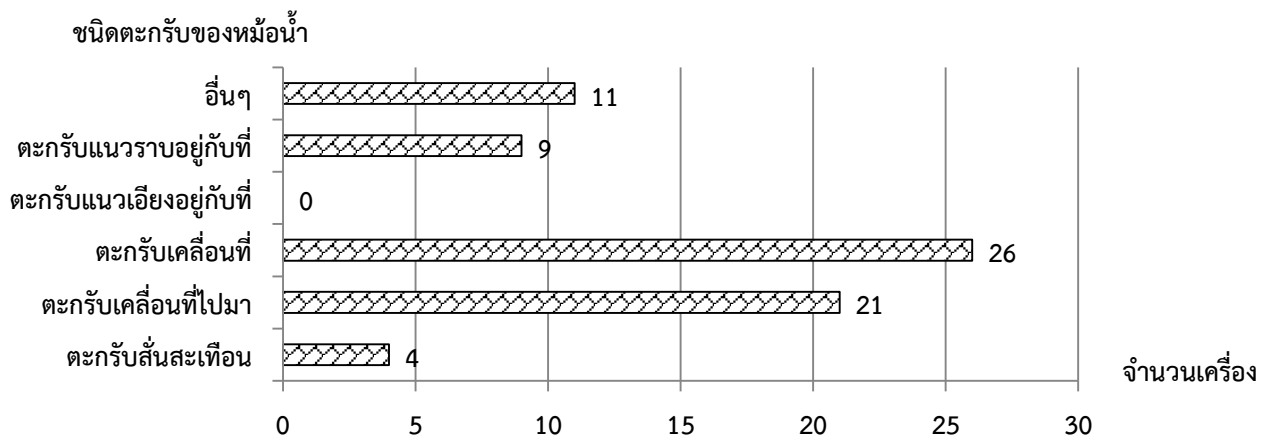
รูปที่ 1.10 ชนิดตะกรับของหม้อน้ำในโรงไฟฟ้าชีวมวลขนาดเล็กมาก (ข้อมูลจากแบบสอบถาม 70 โรงไฟฟ้า)
