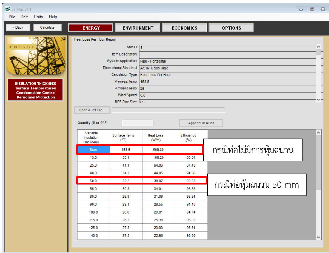
รูปที่ 5.12 ผลการคำนวณความร้อนสูญเสียผ่านผิวท่อด้วยโปรแกรม 3E Plus
