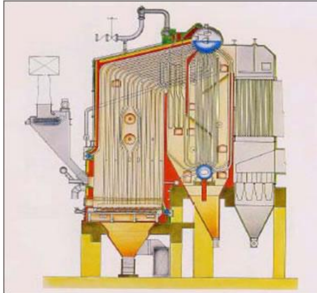
รูปที่ 3.7 ตะกรับเตาแนวราบอยู่กับที่ (Stationary fixed flat grate)
