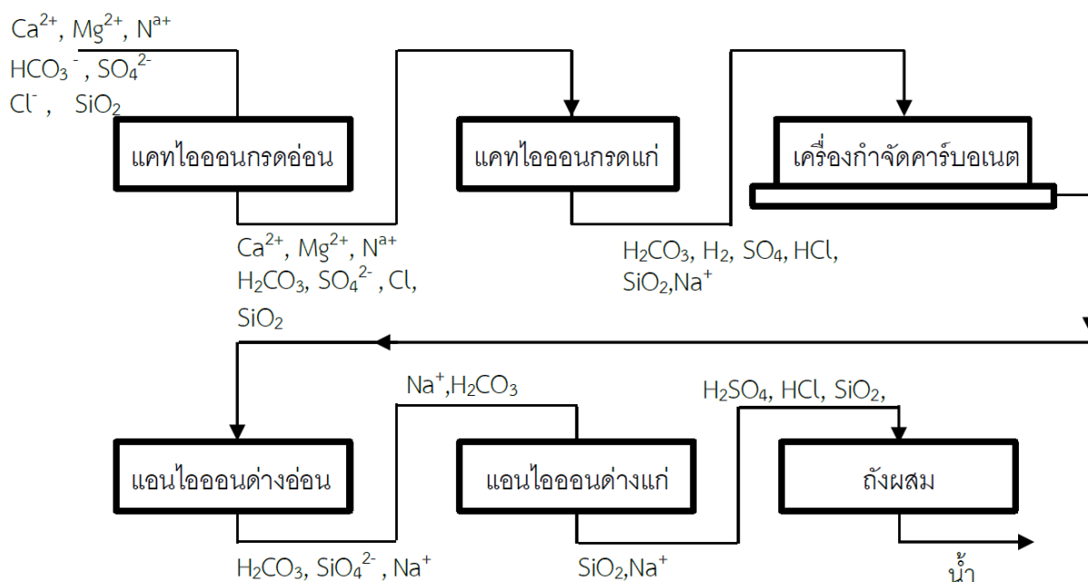
รูปที่ 4.8 กระบวนการปรับสภาพน้ำโดยวิธีแลกเปลี่ยนไอออน [Nag, P.K., 2008]
