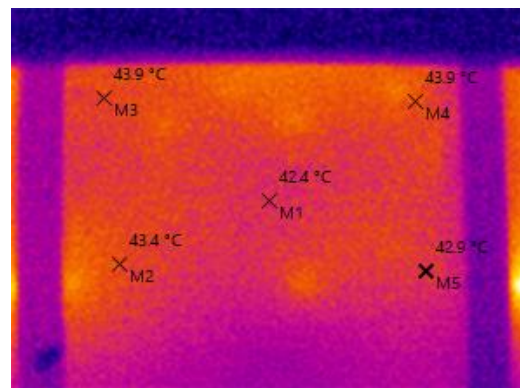
(ง) ภาพถ่ายความร้อนผนังด้านหน้าหม้อน้ำ
