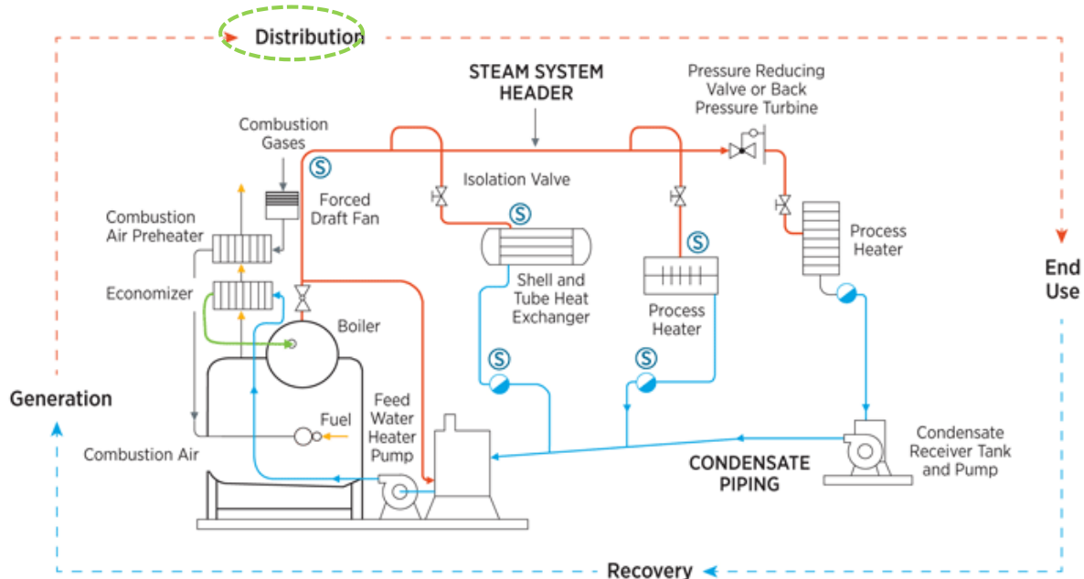
รูปที่ 5.1 ระบบท่อส่งจ่ายไอน้ำ (Steam distribution) เส้นประวงรีสีเขียว
