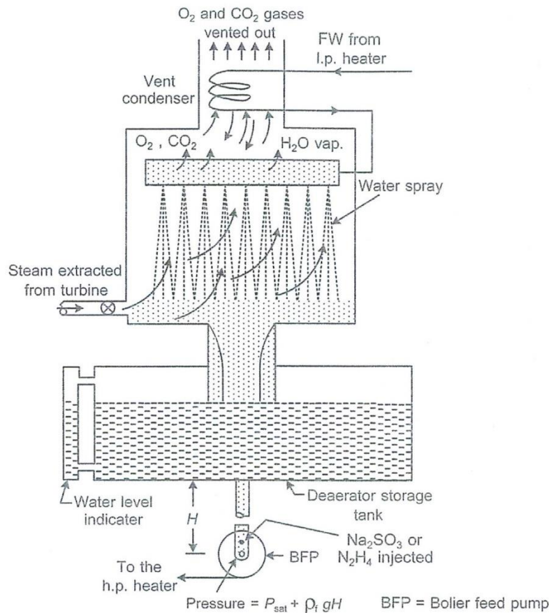
รูปที่ 2.6 เครื่องกำจัดฟองอากาศ (Deaerator)
