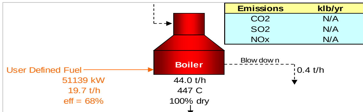
รูปที่ 9.30 แบบจำลองจากการปรับปรุงประสิทธิภาพอุปกรณ์อุ่นน้ำป้อนหม้อน้ำด้วยโปรแกรม SSAT
