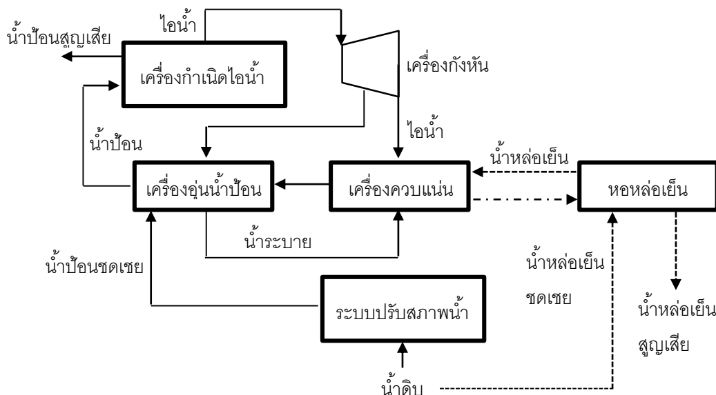
รูปที่ 7.1 ระบบน้ำป้อนและน้ำหล่อเย็น
