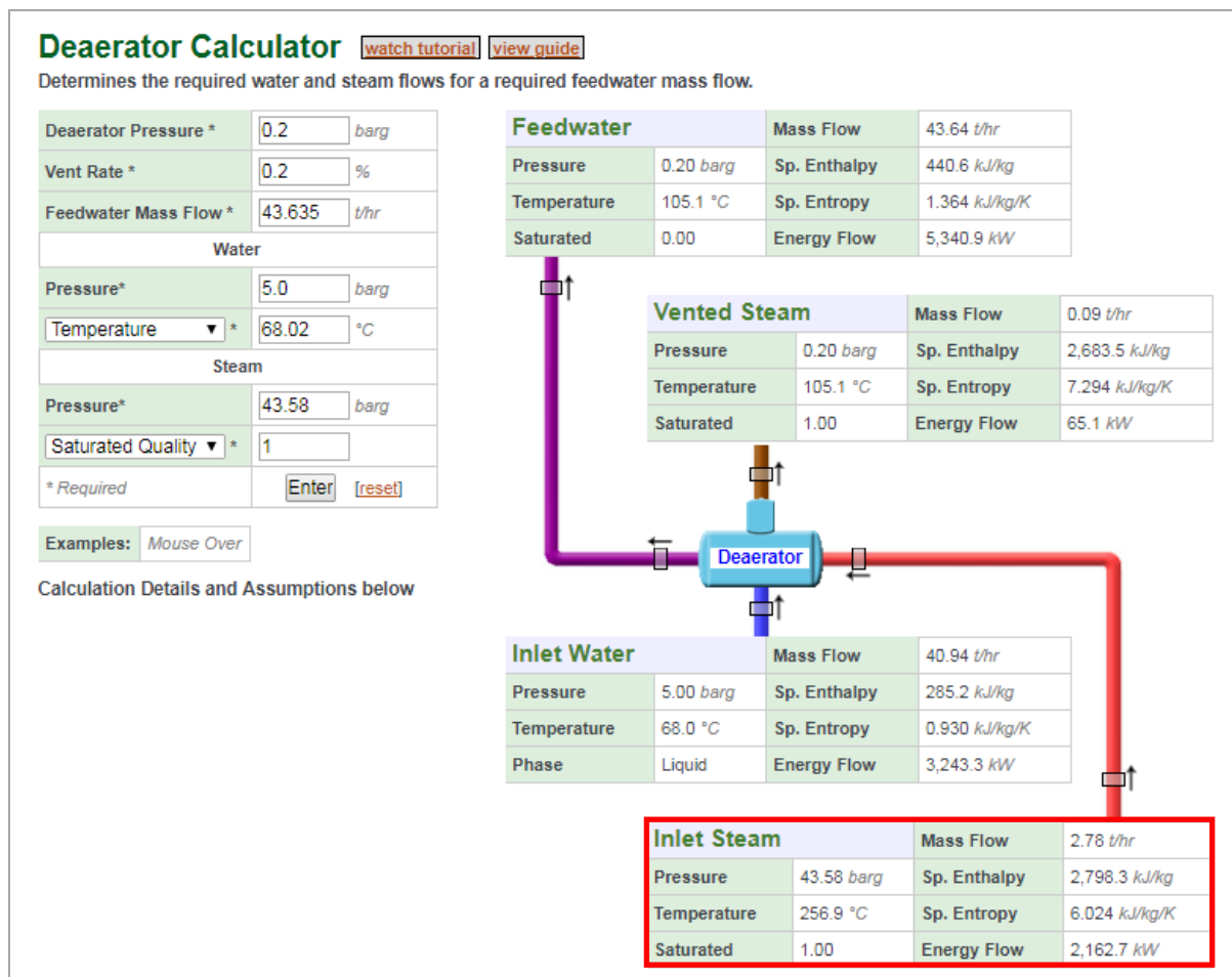
รูปที่ 9.49 การคำนวณปริมาณไอน้ำจากดรัมบนที่ใช้อุ่นน้ำในดีแอรเรเตอร์ (ก่อนการปรับปรุง)
