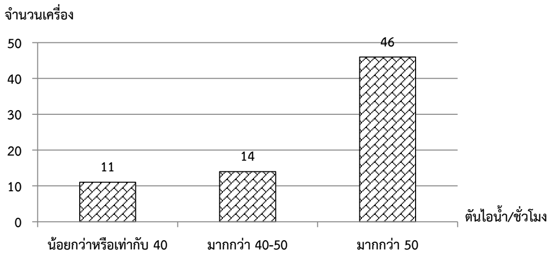
รูปที่ 1.8 ขนาดพิกัดหม้อน้ำในโรงไฟฟ้าชีวมวลขนาดเล็กมาก (ข้อมูลจากแบบสอบถาม 70 โรงไฟฟ้า)
