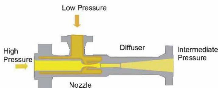
รูปที่ 1.23 Steam-jet air ejector
