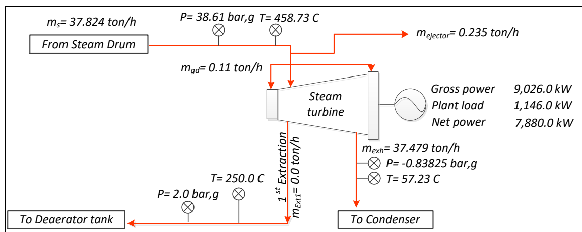
รูปที่ 9.62 ไดอะแกรมการใช้ไอน้ำหลังการปรับปรุงมาตรการลดความดันไอน้ำขาออกจากกังหันไอน้ำ
