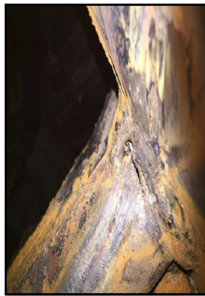
รูปที่ 10.3 Boiler Tube Leak ที่แนวเชื่อมต่อ Back Water Wall Tube กับ Upper Header
