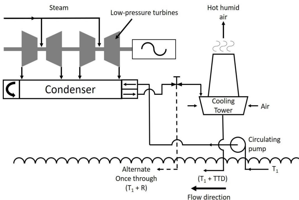
รูปที่ 8.3 ระบบน้ำหล่อเย็นแบบเปิดทำงานร่วมกันแบบปิด
