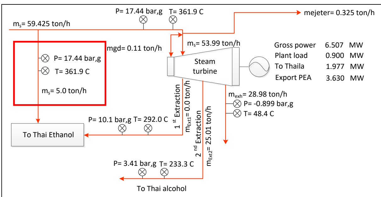
รูปที่ 9.69 ไดอะแกรมการใช้ไอน้ำ ณ วันที่เข้าตรวจวัดกังหันไอน้ำ (ก่อนปรับปรุง)
