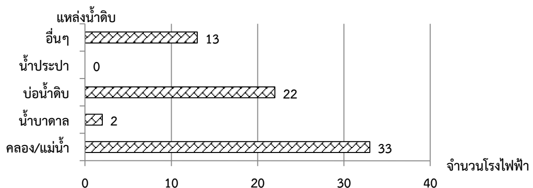
รูปที่ 1.14 แหล่งน้ำดิบสำหรับโรงไฟฟ้าชีวมวลขนาดเล็กมาก (ข้อมูลจากแบบสอบถาม 70 โรงไฟฟ้า)
