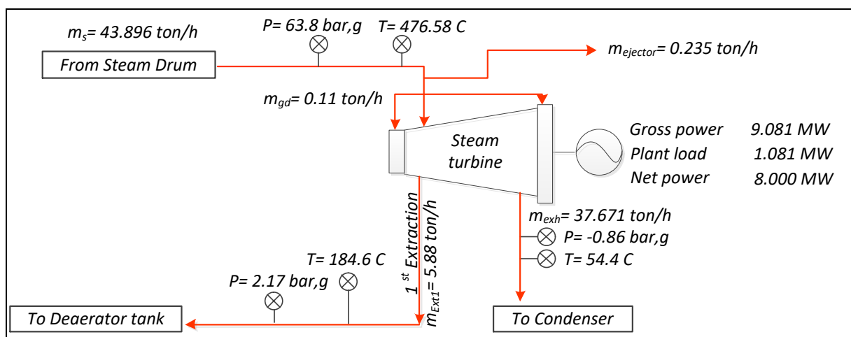
รูปที่ 9.86 ไดอะแกรมการใช้ไอน้ำจากมาตรการปรับลดขายไฟ PEA เหลือขาย 8.0 MW ตามสัญญา (หลังการปรับลดไอน้ำที่ใช้ในการผลิตไฟฟ้า)
