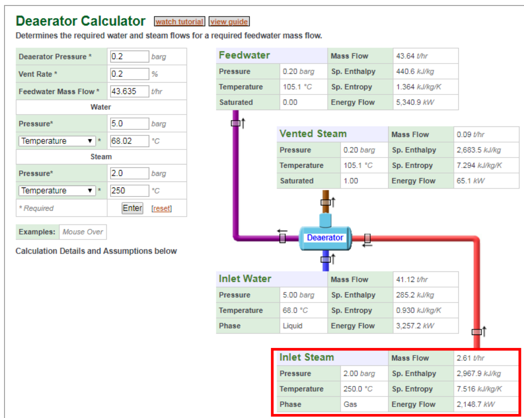
รูปที่ 9.52 การคำนวณปริมาณไอน้ำแรงดันต่ำจากกังหันไอน้ำที่ใช้อุ่นน้ำในดีแอร์เรเตอร์ (หลังการปรับปรุง)
