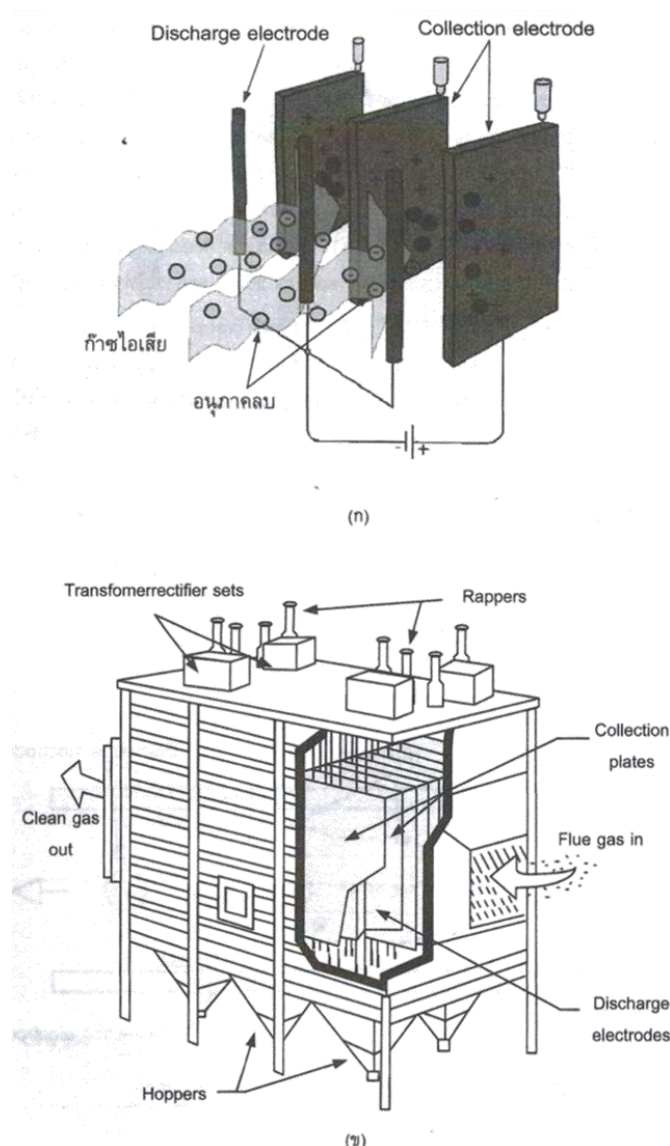
รูปที่ 3.19 (ก) การดักจับฝุ่นภายในเครื่องดักฝุ่นแบบไฟฟ้าสถิต (ESP) และ (ข) เครื่องดักฝุ่นแบบไฟฟ้าสถิต (ESP)
