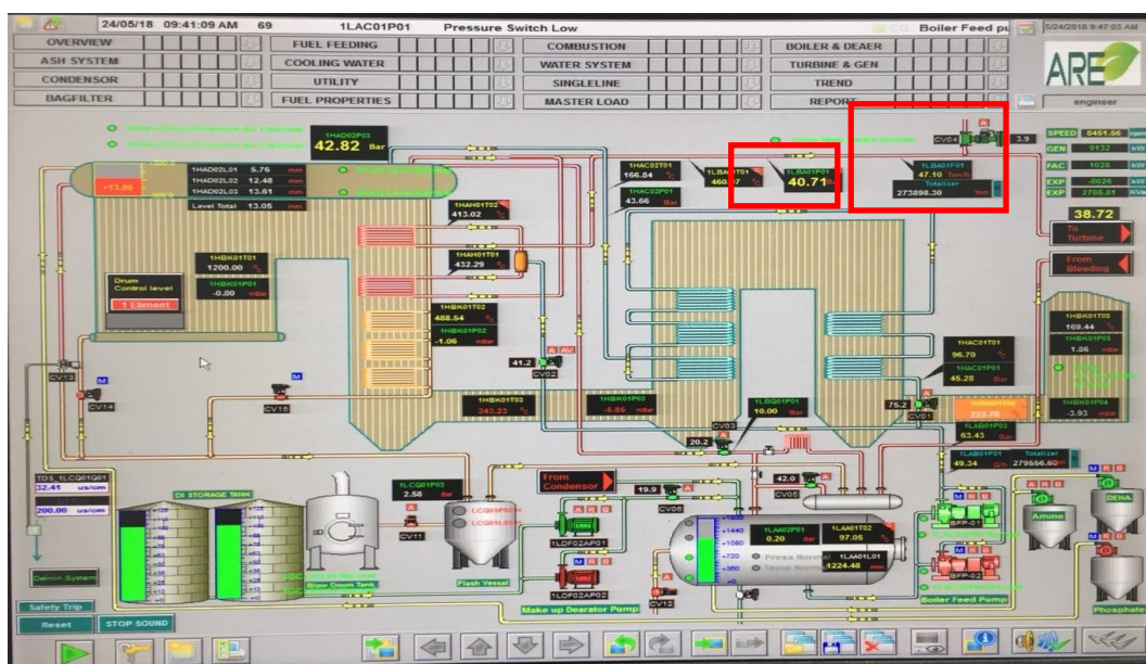
รูปที่ 9.6 จอแสดง Boiler main steam pressure และ Boiler startup vent valve control
