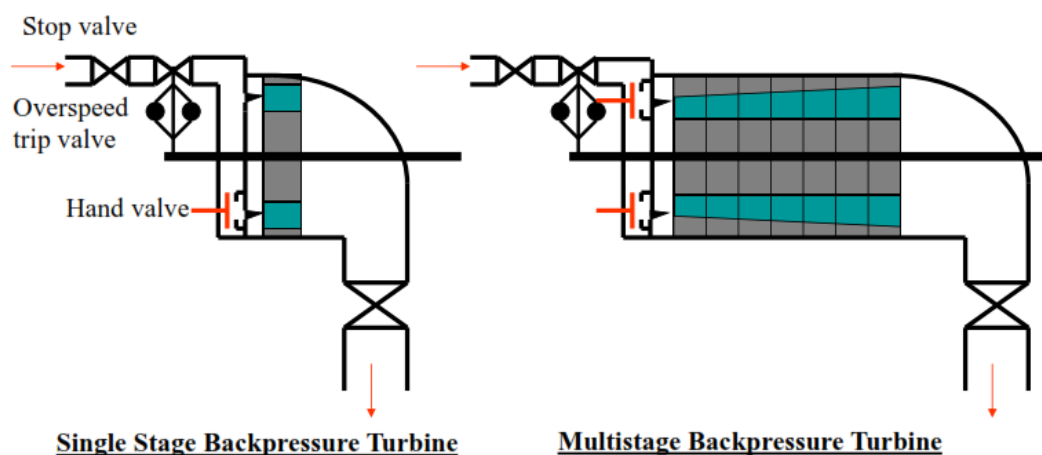
รูปที่ 6.2 (b) แผงผังของ Back pressure turbine
