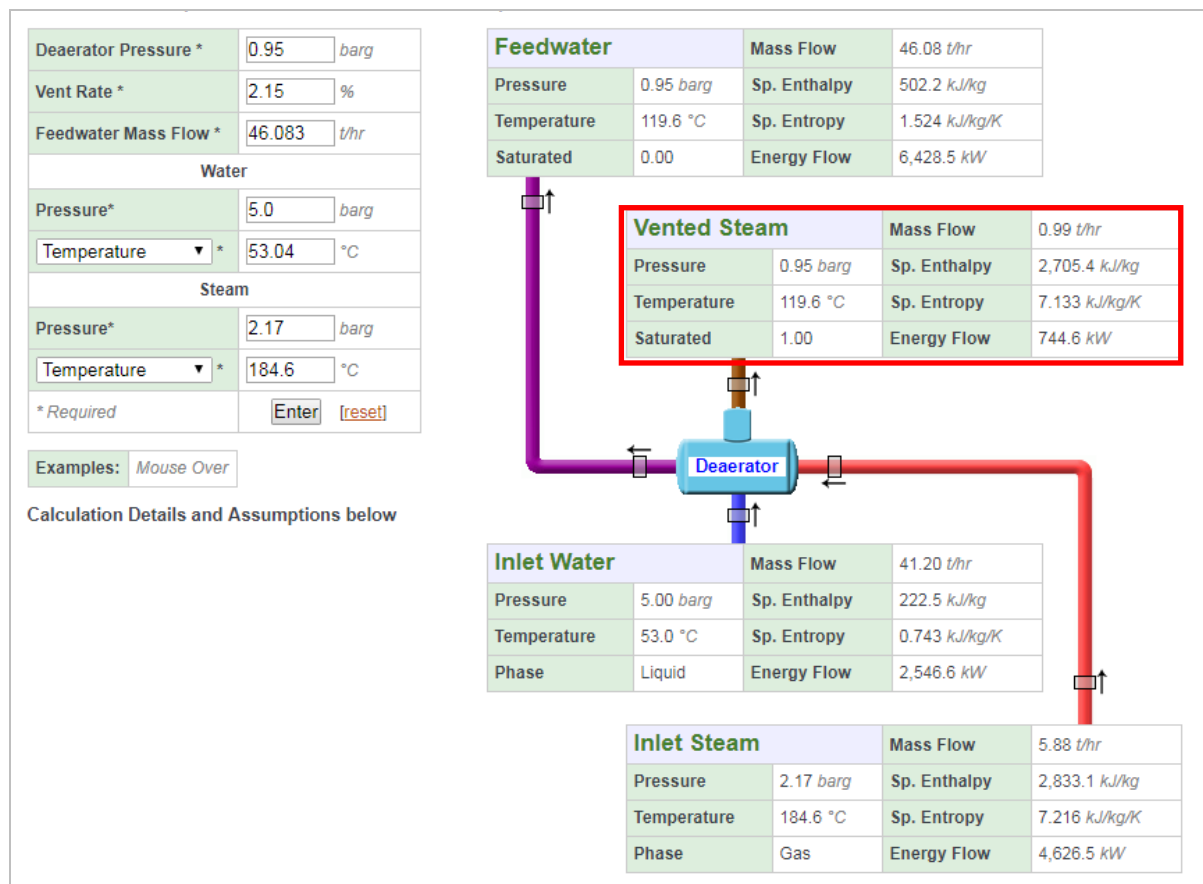
รูปที่ 9.41 การประเมินการใช้ไอน้ำอุ่นน้ำป้อนในถังดีแอเรเตอร์ และปริมาณ Vent out (ก่อนปรับปรุง)
