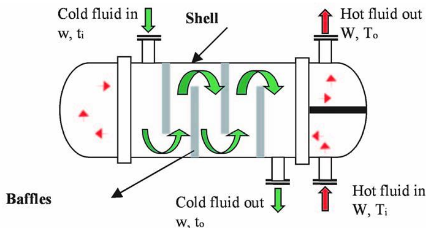
รูปที่ 7.10 หลักการแลกเปลี่ยนความร้อนของเครื่องแลกเปลี่ยนความร้อนแบบเปลือกและท่อ
