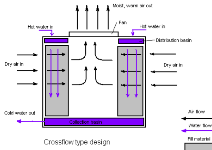
(บ) แผนภาพหอผึ่งเย็นแบบไหลตามขวาง
