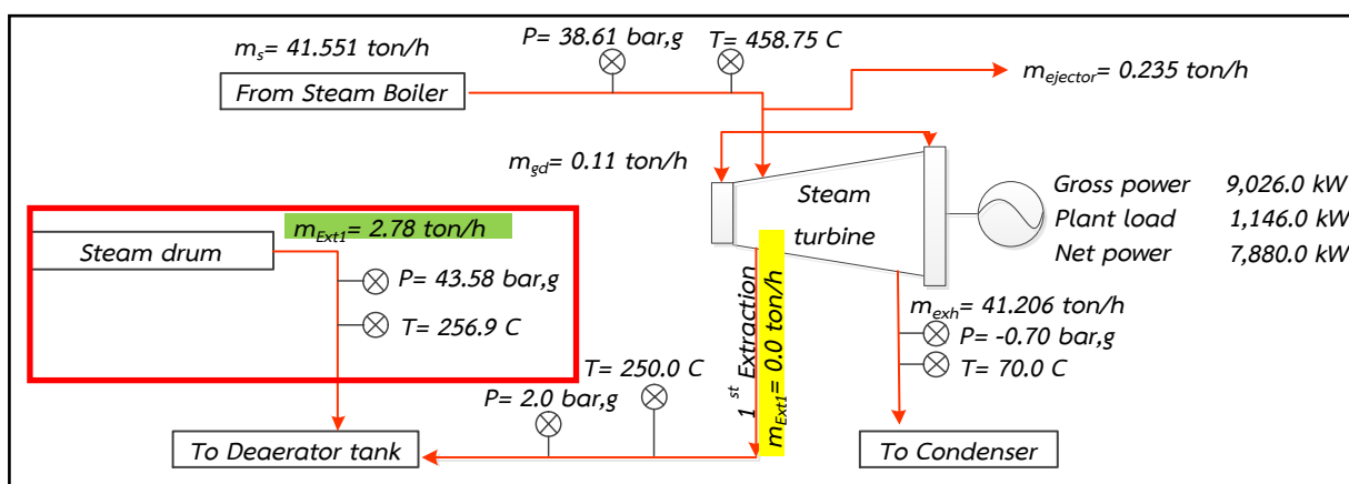
รูปที่ 9.48 แผนผังการใช้ไอน้ำในดีเออร์เรเตอร์ (ก่อนการปรับปรุง)
