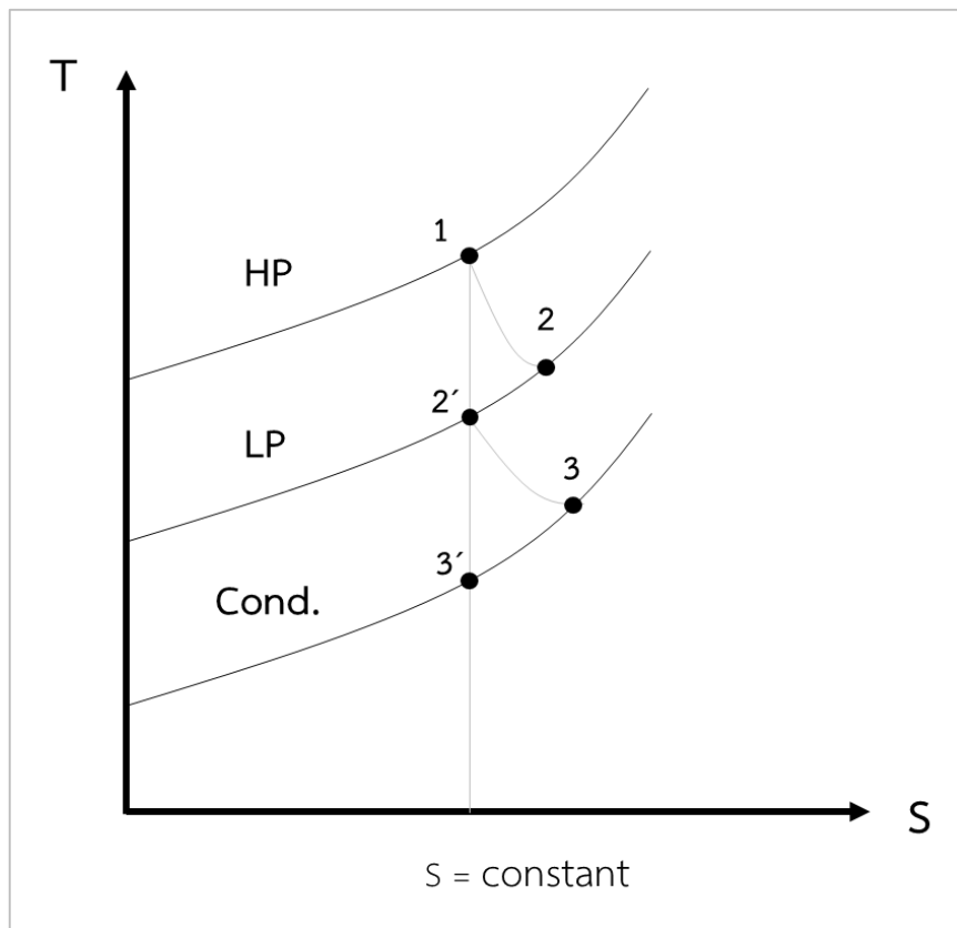
รูปที่ 6.30 เกณฑ์การหาประสิทธิภาพไอเซนโทรปิกของกังหันไอน้ำ
